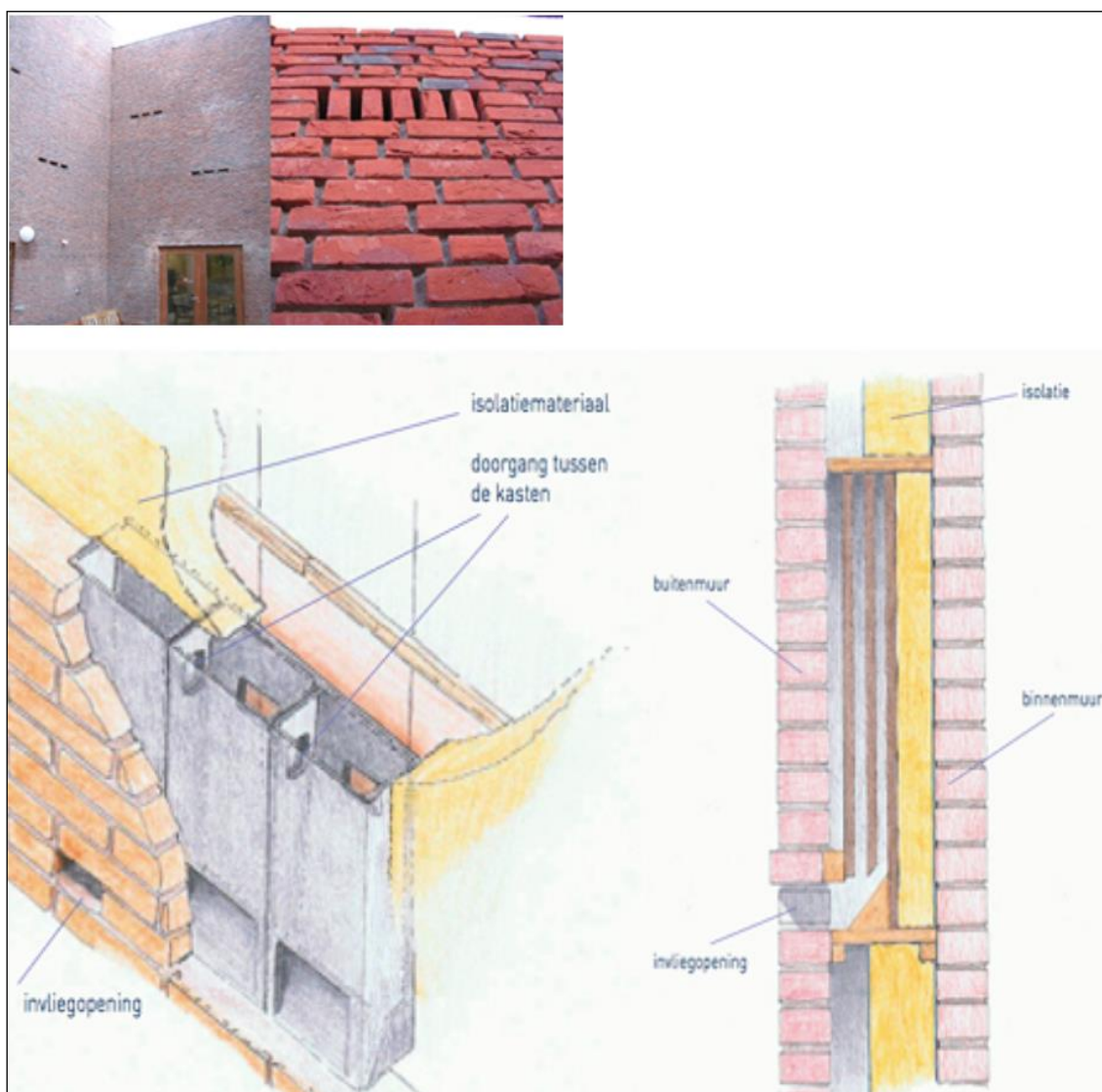
Figuur 7: Vrijwel onzichtbare inbouw van vleermuisstenen en technische informatie over de plaatsing daarvan
