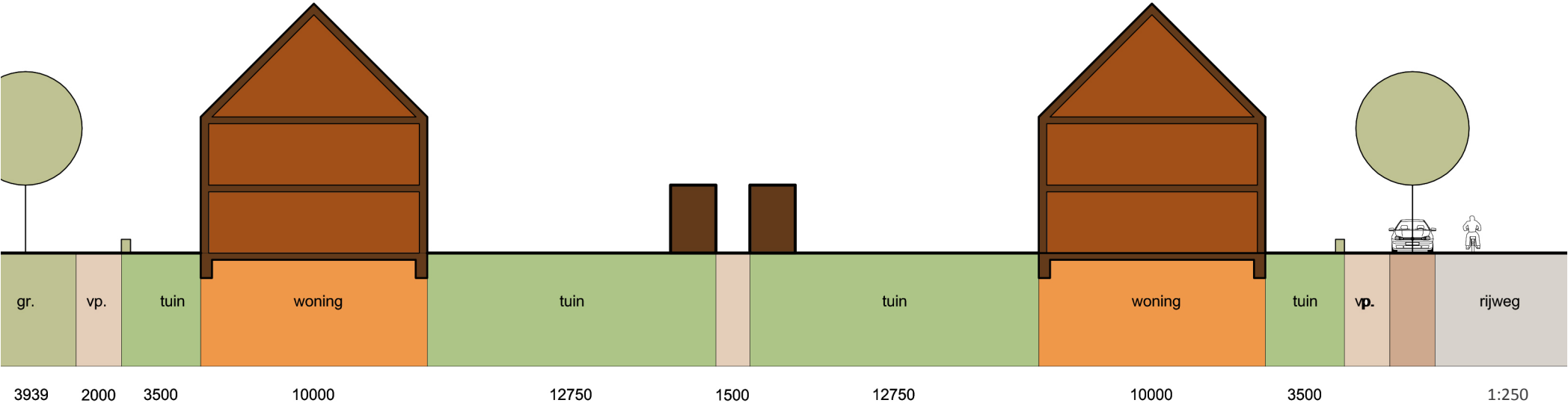
Profiel B - woonstraat - Eengezinswoningen
