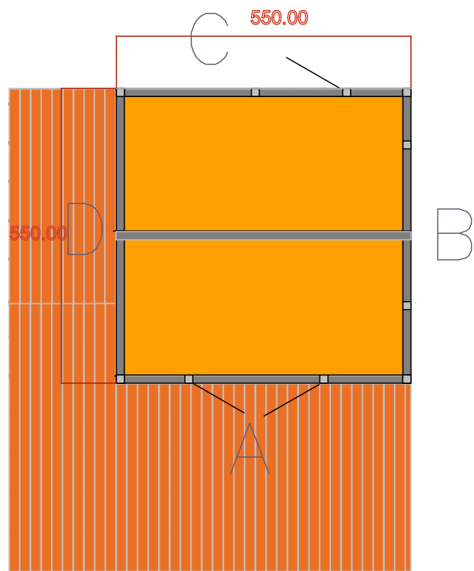
Hardhouten vlonder 2.8*19 cm buiten Douglas vlonder 2.8*19 binnen
