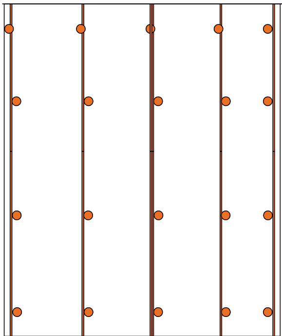
funderingsplan vlonder. geïmpregneerde paal 10 * 500 cm
