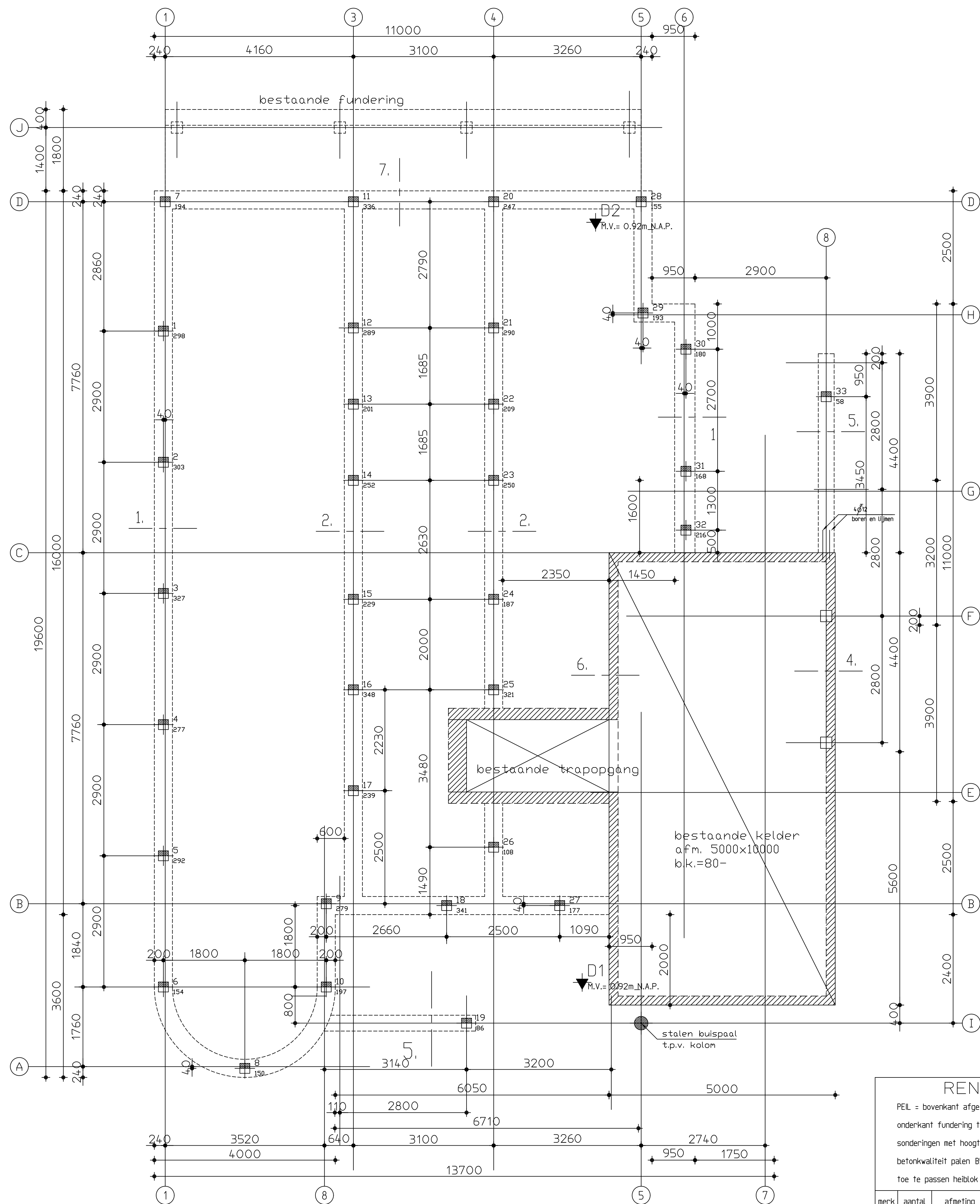
MAATV. FUNDERING
