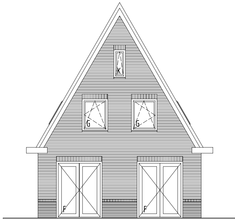
Westgevel
