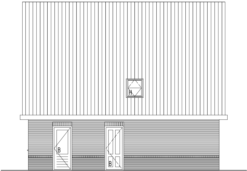
Noordgevel
