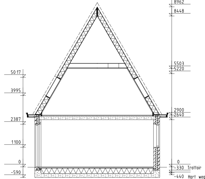
Doorsnede
