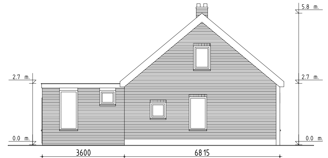
Zuidgevel
