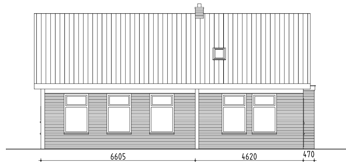
Oostgevel
