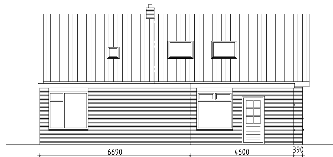
Westgevel
