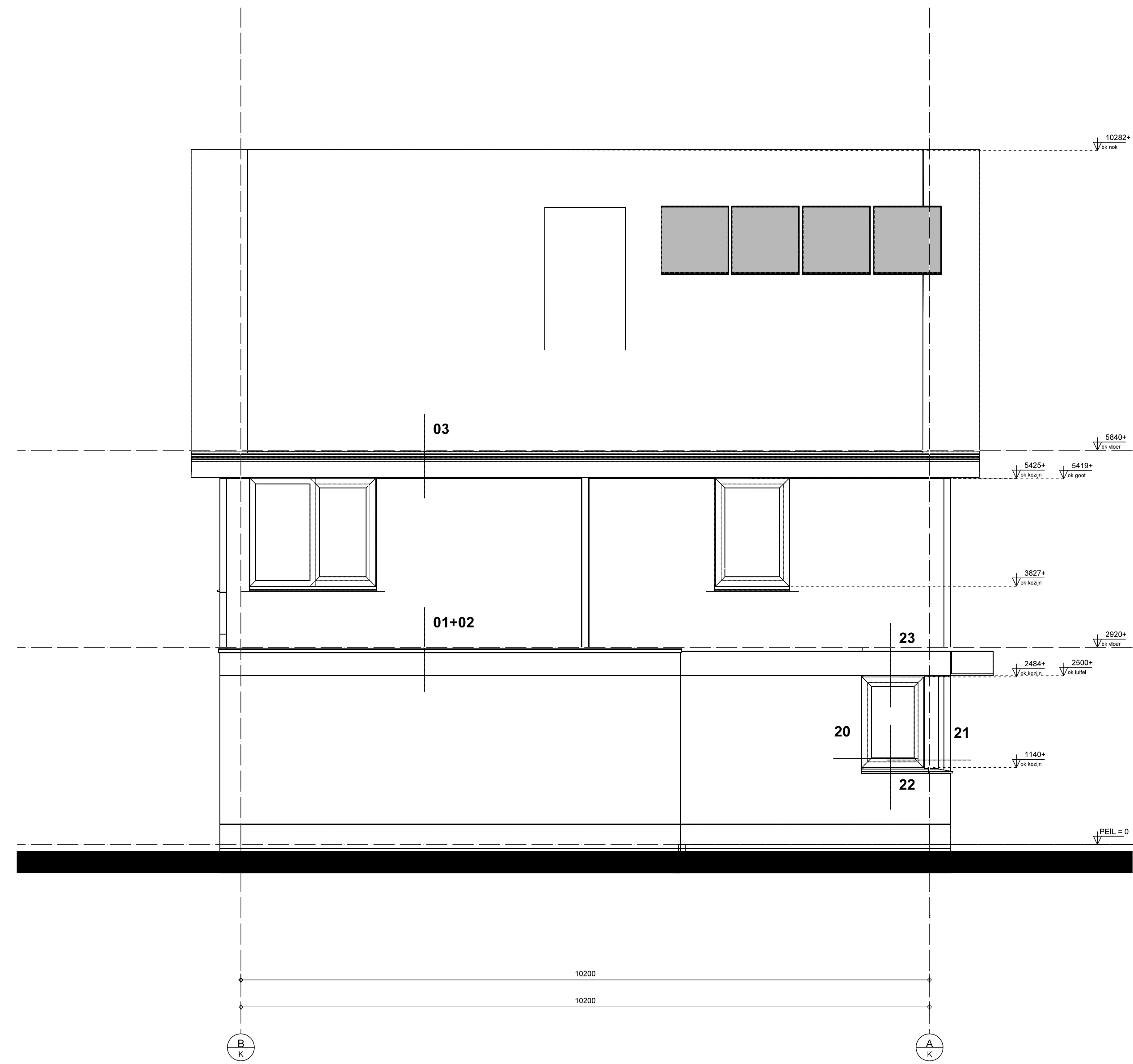
LINKERZIJGEVEL
