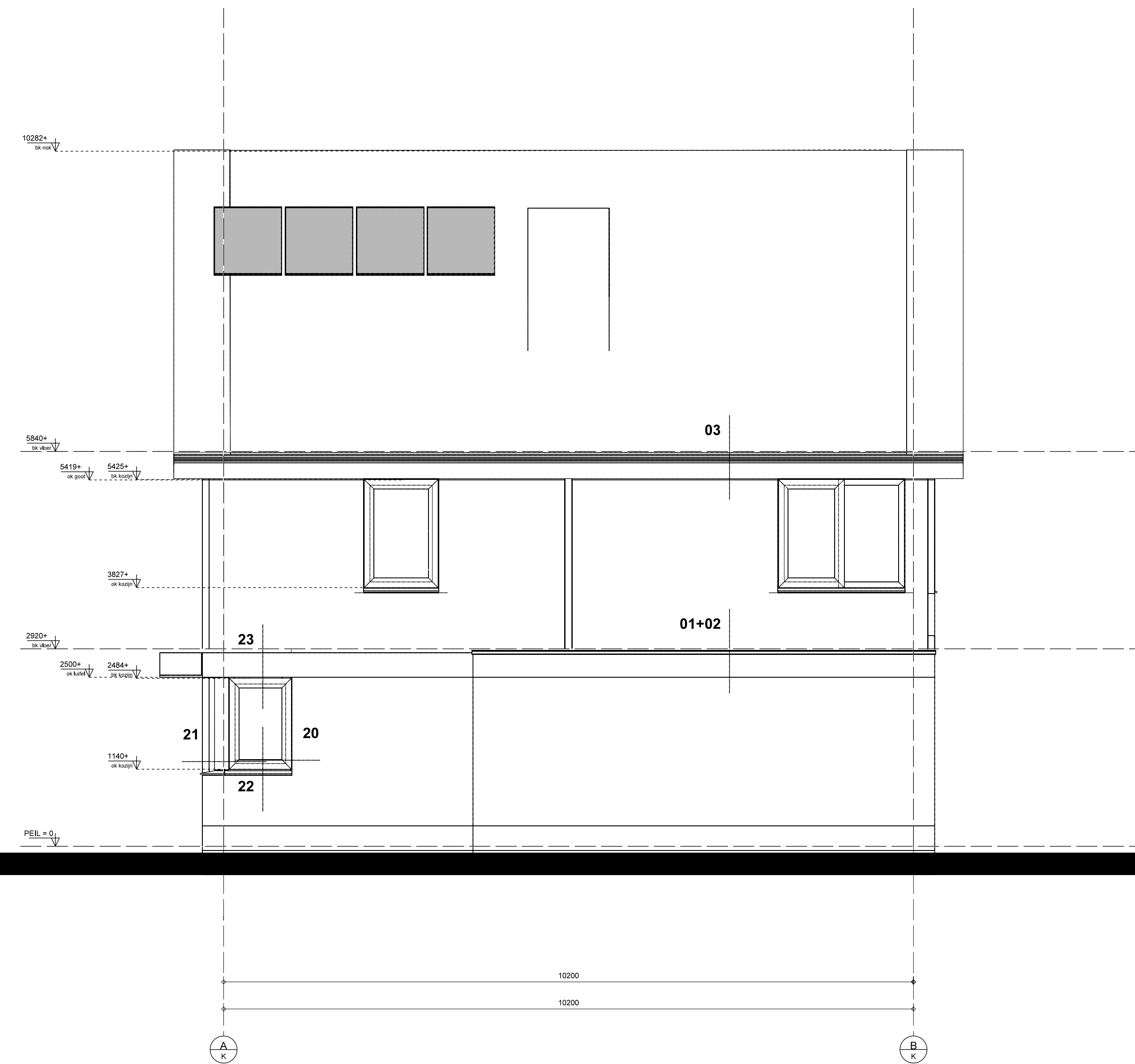
RECHTERZIJGEVEL
