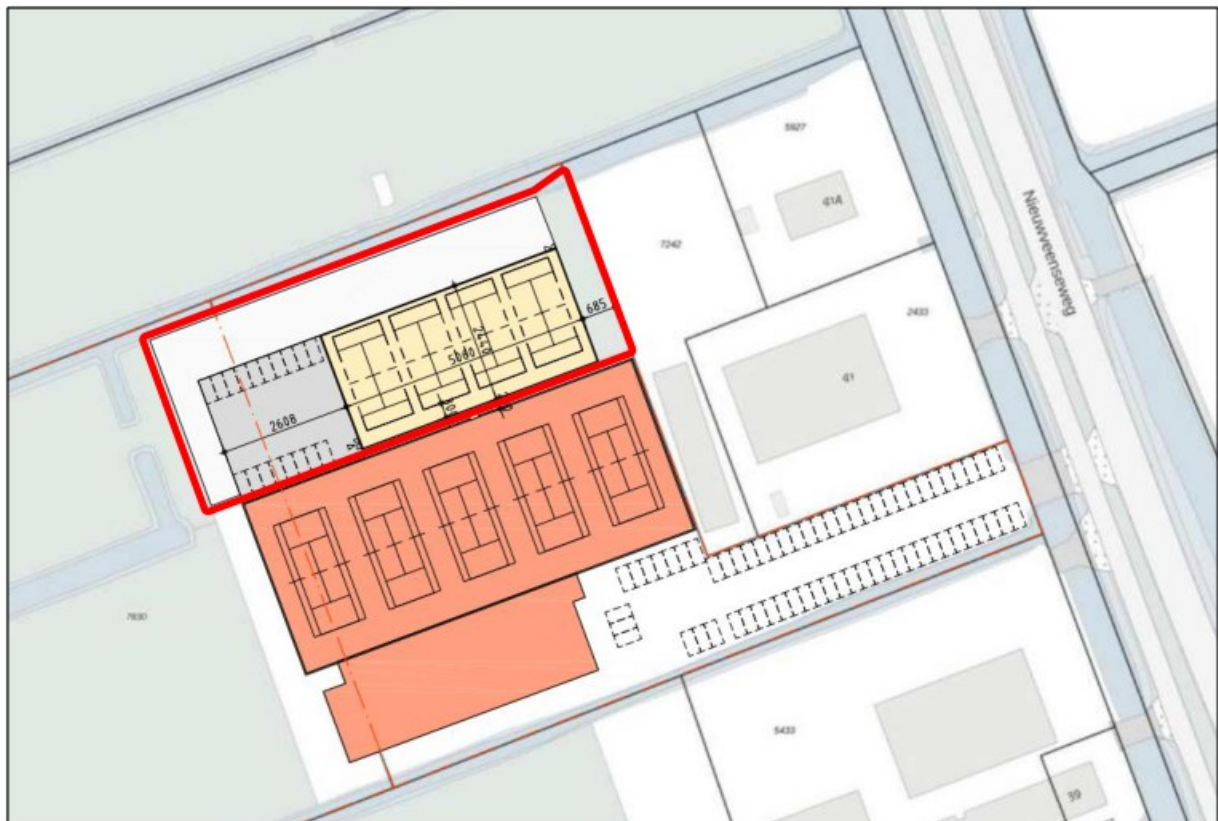
Figuur 17. Voorlopig ontwerp padelhal en parkeerterrein.
