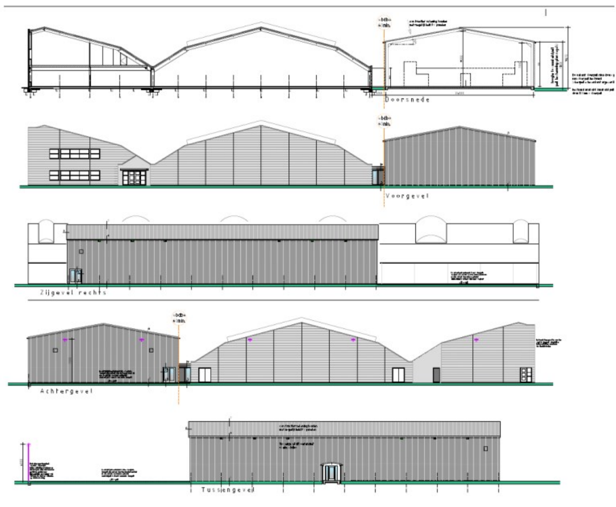
Figuur 7: definitief ontwerp padelhal architect
