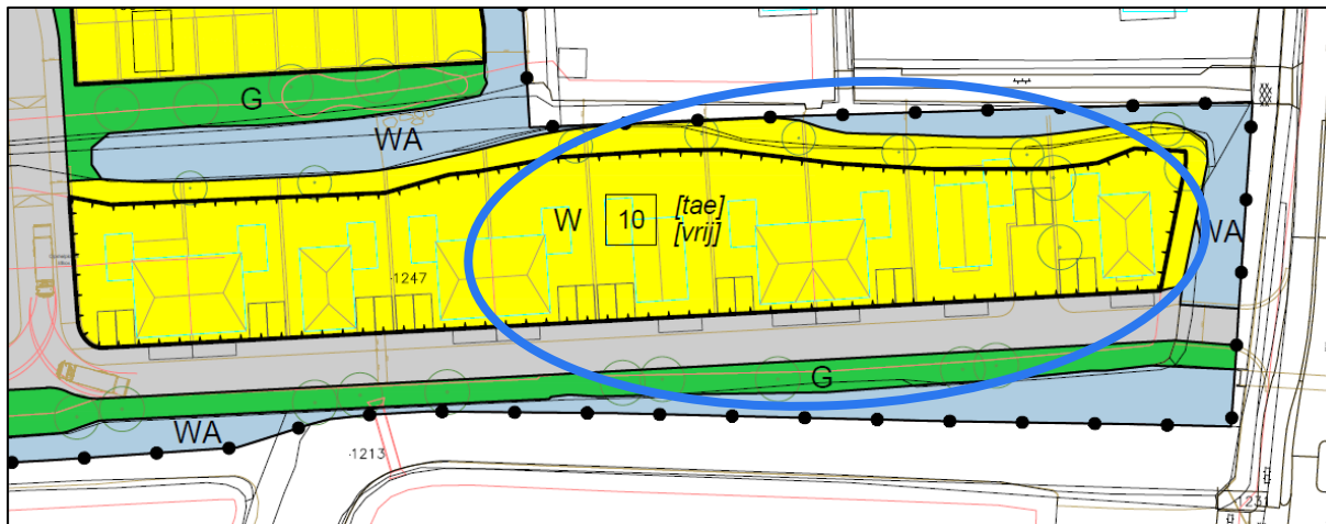
afbeelding 3: planvoornemen
