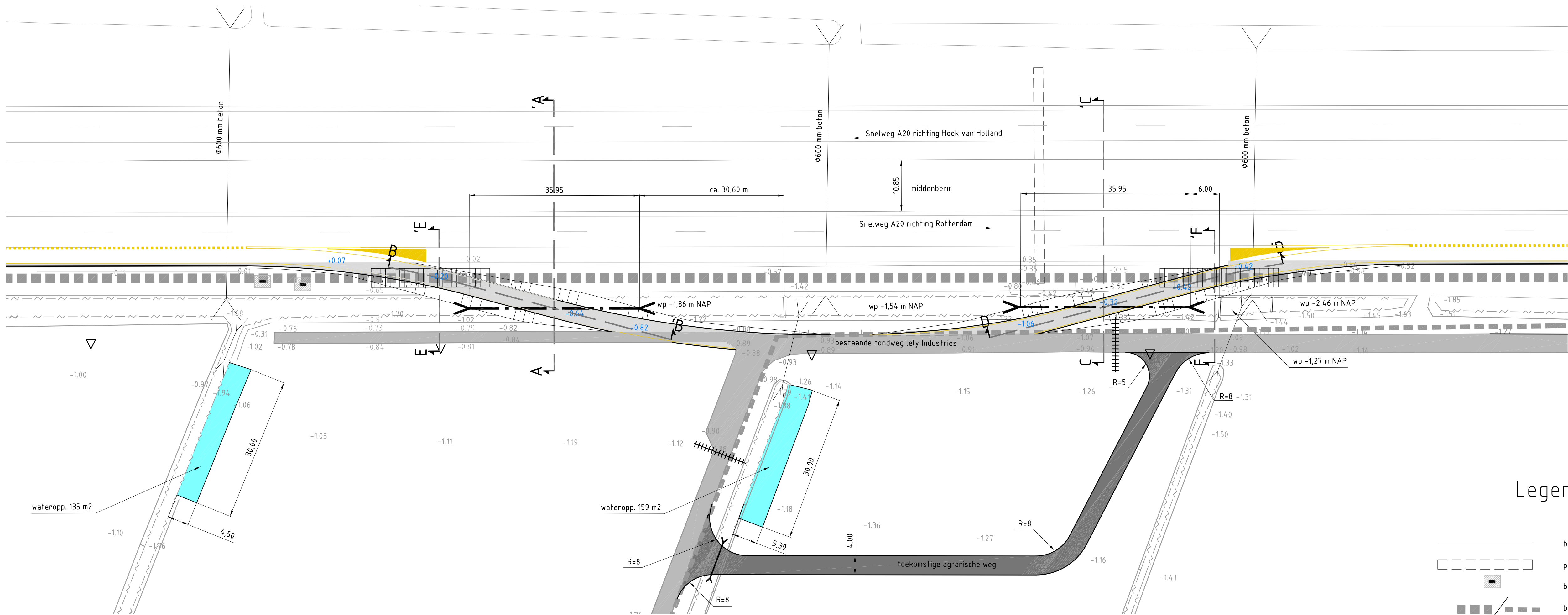
Uitsnede 1: tijdelijke af- en oprit A20 schaal 1:500
