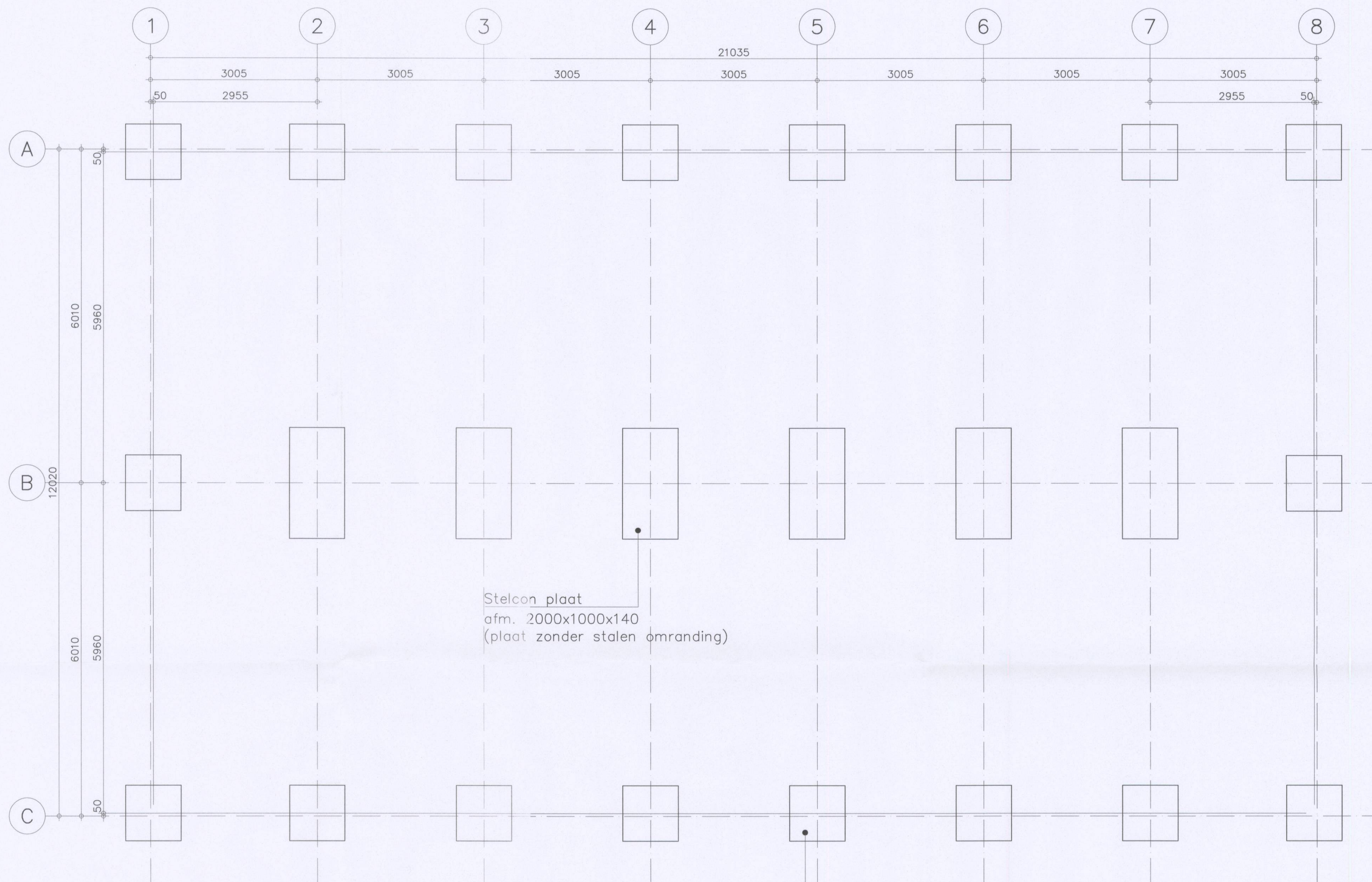
OVERZICHT FUNDATIE (Stelcon platen) Schaal 1:50
