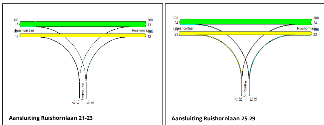
Figuur 3.2: Verkeersstromen drukste uur (17.00-18.00 uur)
