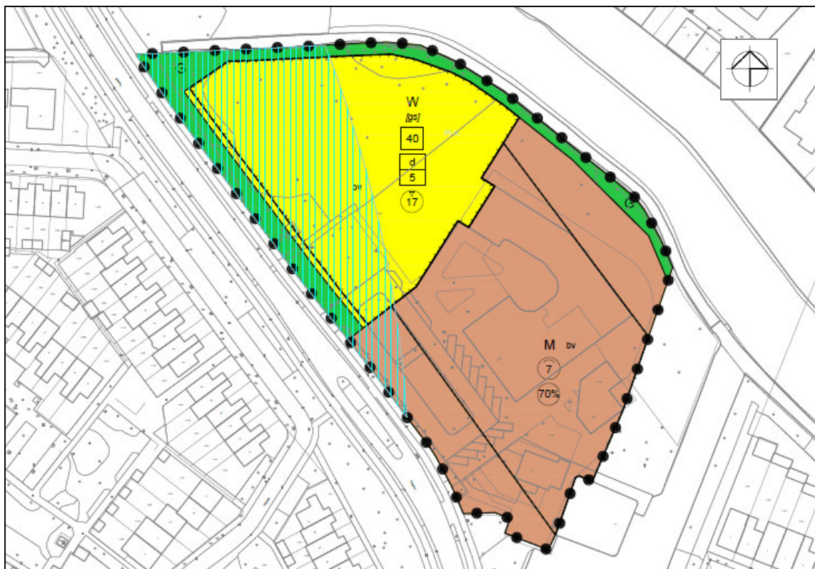
Figuur 1.3: Plankaart Ruishornlaan 25 in Lisse (bron: Wissing)
