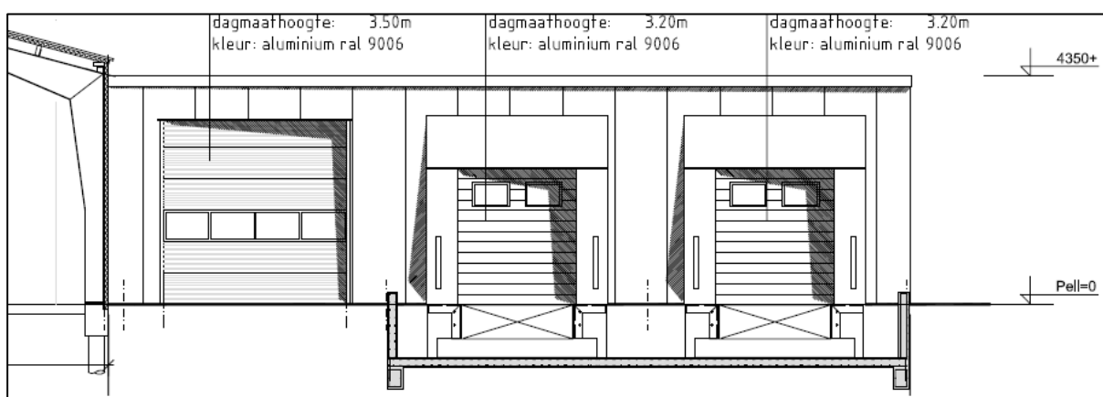
Figuur 1: Detail van de zuid-west gevel van de geplande nieuwbouw, met rechts het laaddock en helemaal links de nieuwe loods.
