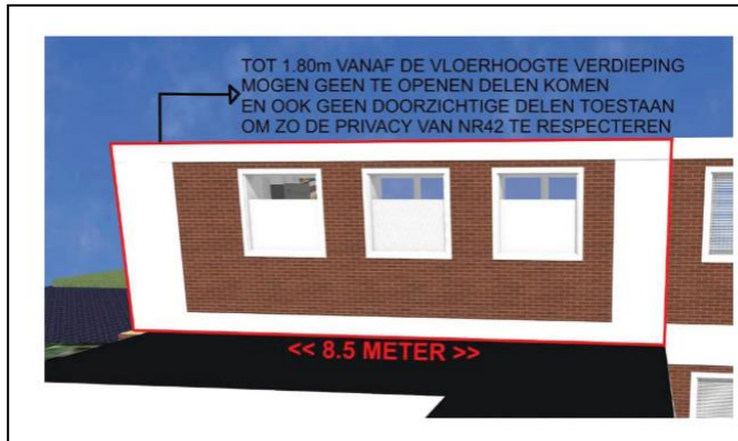
Afbeelding: weergegeven is een maatregel ten behoeve van het borgen van de privacy op het buurperceel Doeslaan 42. In het wijzigingsplan is bepaald dat relevante ramen tot 1,80 meter vanaf de verdiepingsvloer niet doorzichtig mogen zijn. Dit over een lengte van 8,5 meter.
