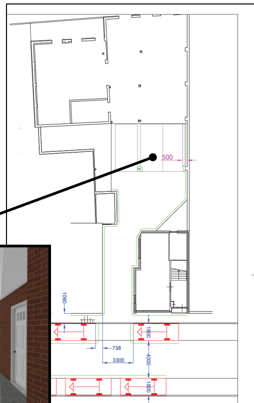
Afbeelding: weergegeven is de begane grond van het projectgebied in de nieuwe situatie. Ter plaatse van het binnenterrein zijn drie parkeerplaatsen voorzien.
