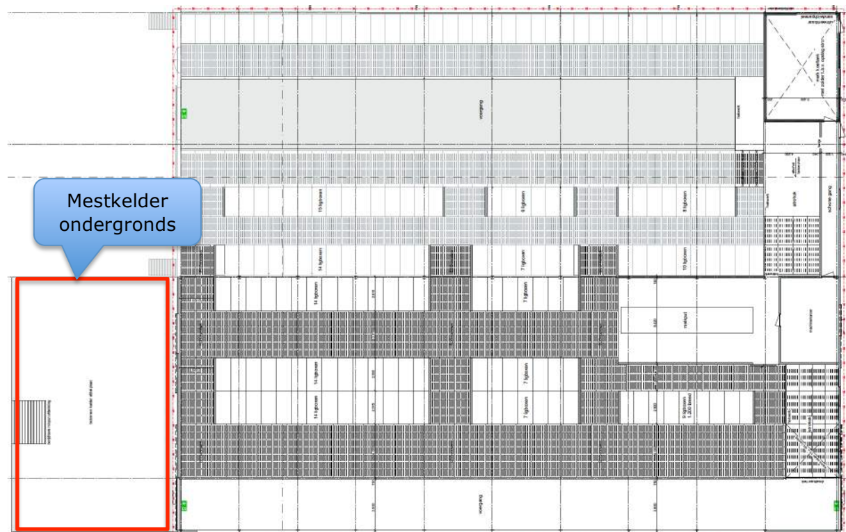
Afbeelding 4.3: Nieuwe ligboxenstal met hierbij verlengde mestkelder ondergronds weergegeven.
