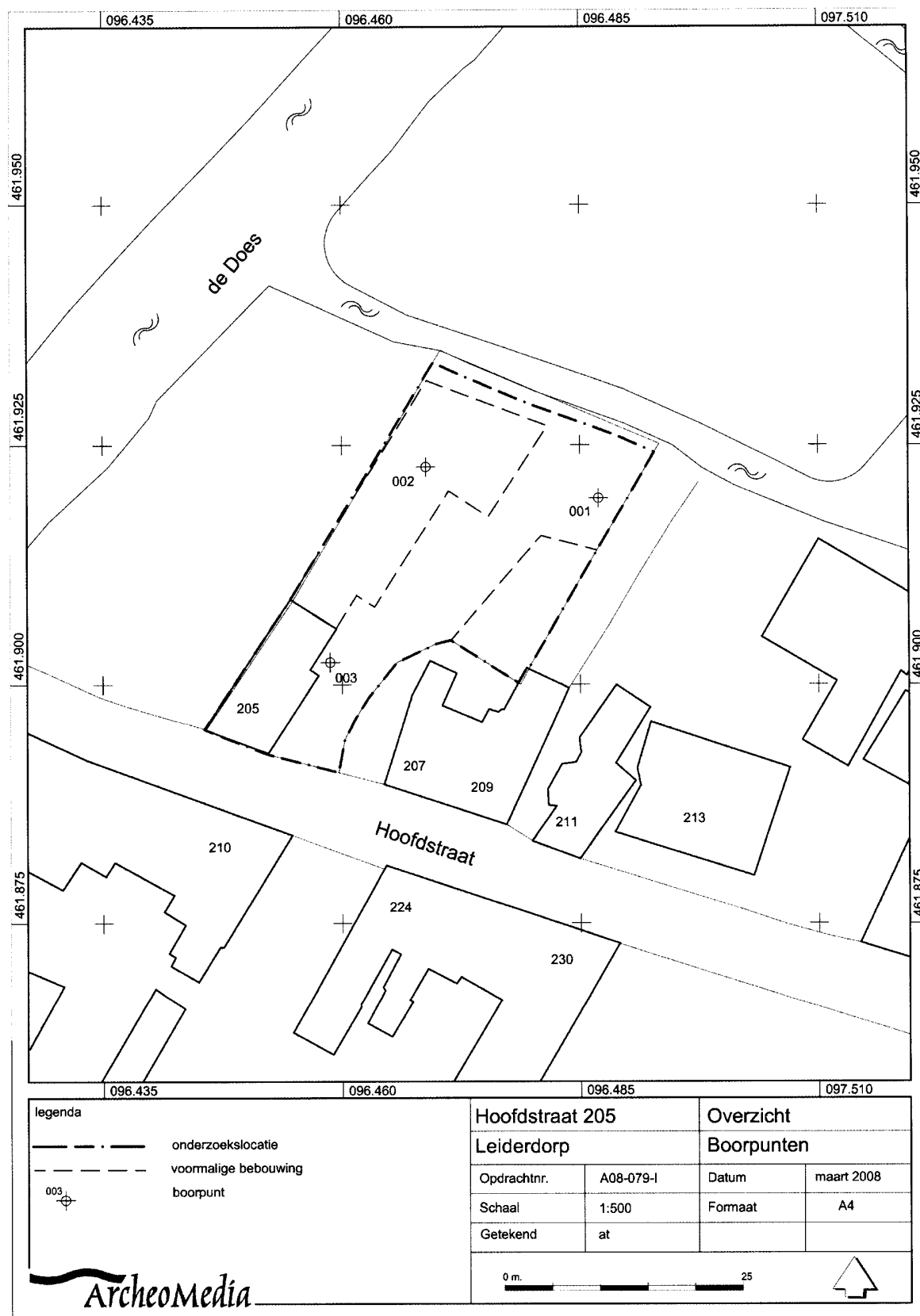
Afbeelding 4: boorpuntenkaart.
