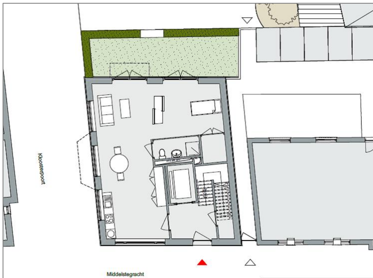
Figuur 3.1 Planindeling
