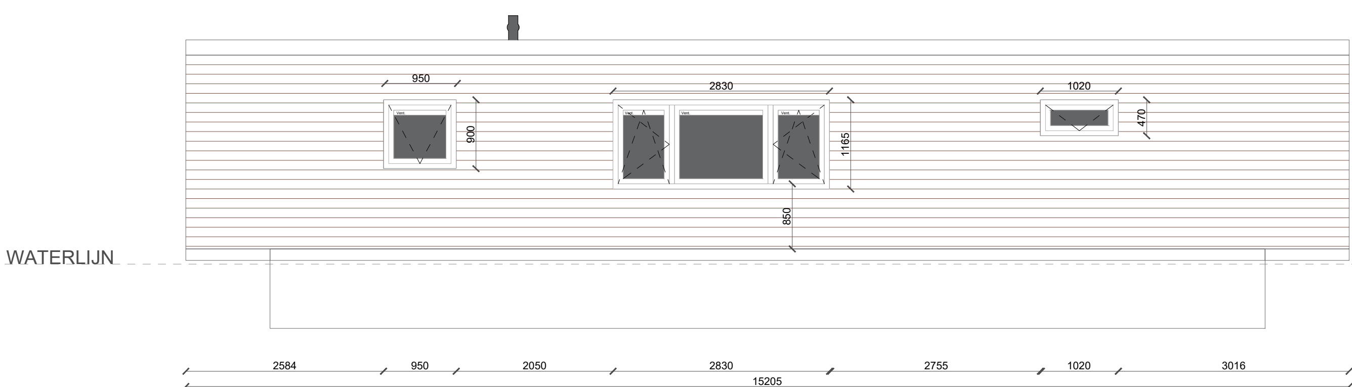
ACHTERGEVEL
