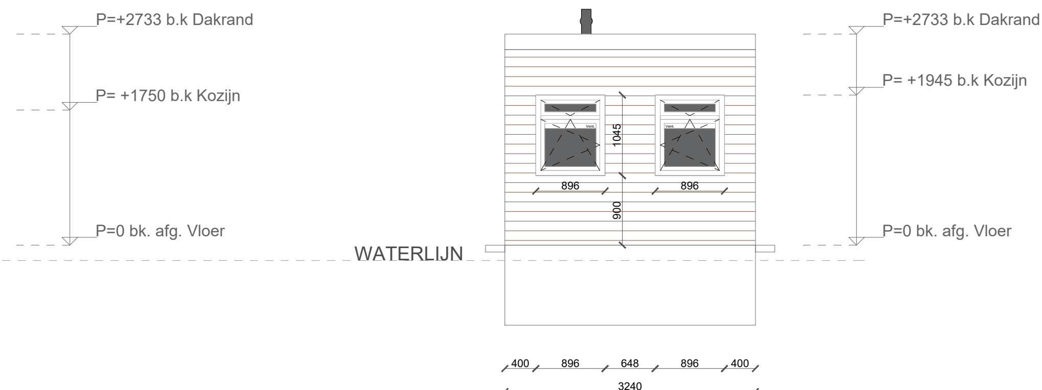
RECHTERZIJGEVEL
