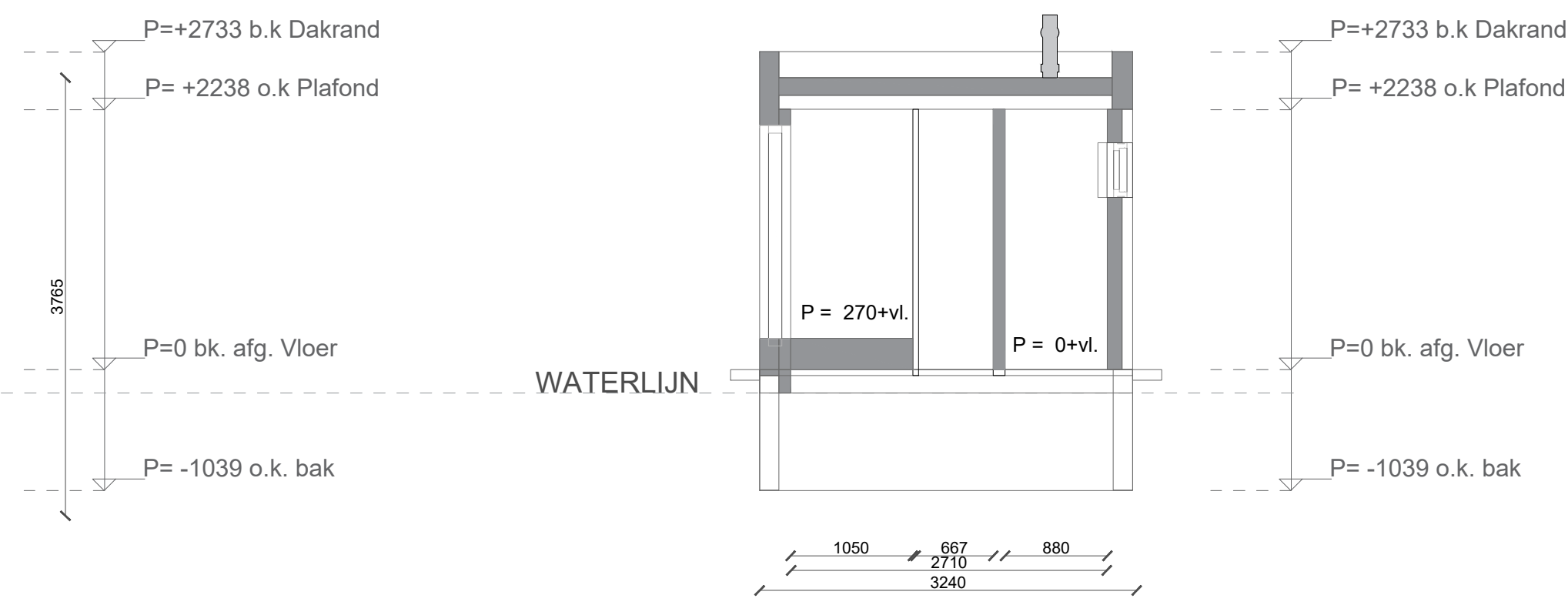
DOORSNEDE BB
