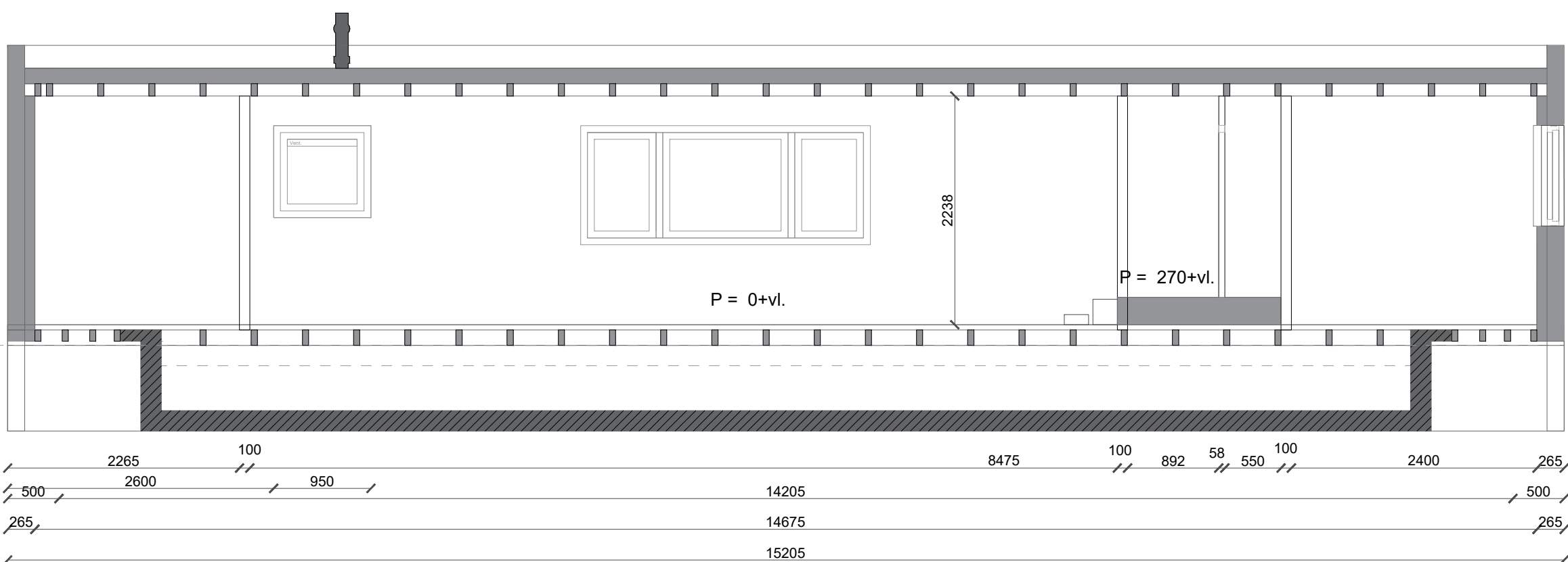
DOORSNEDE AA
