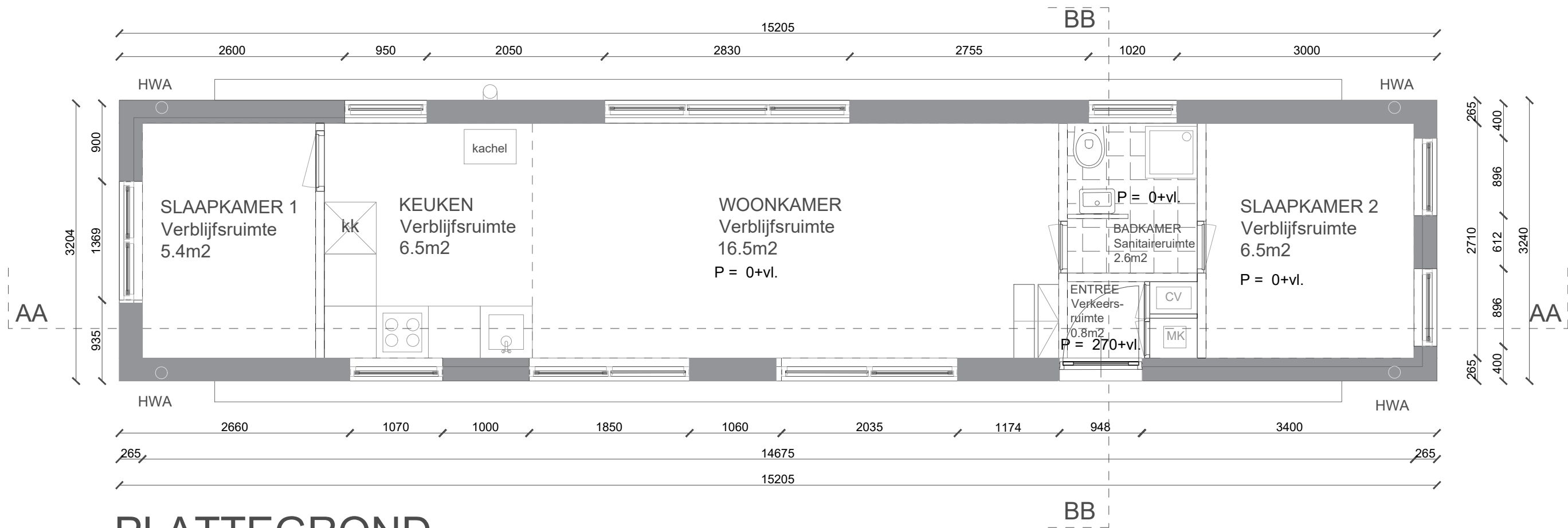
PLATTEGROND
