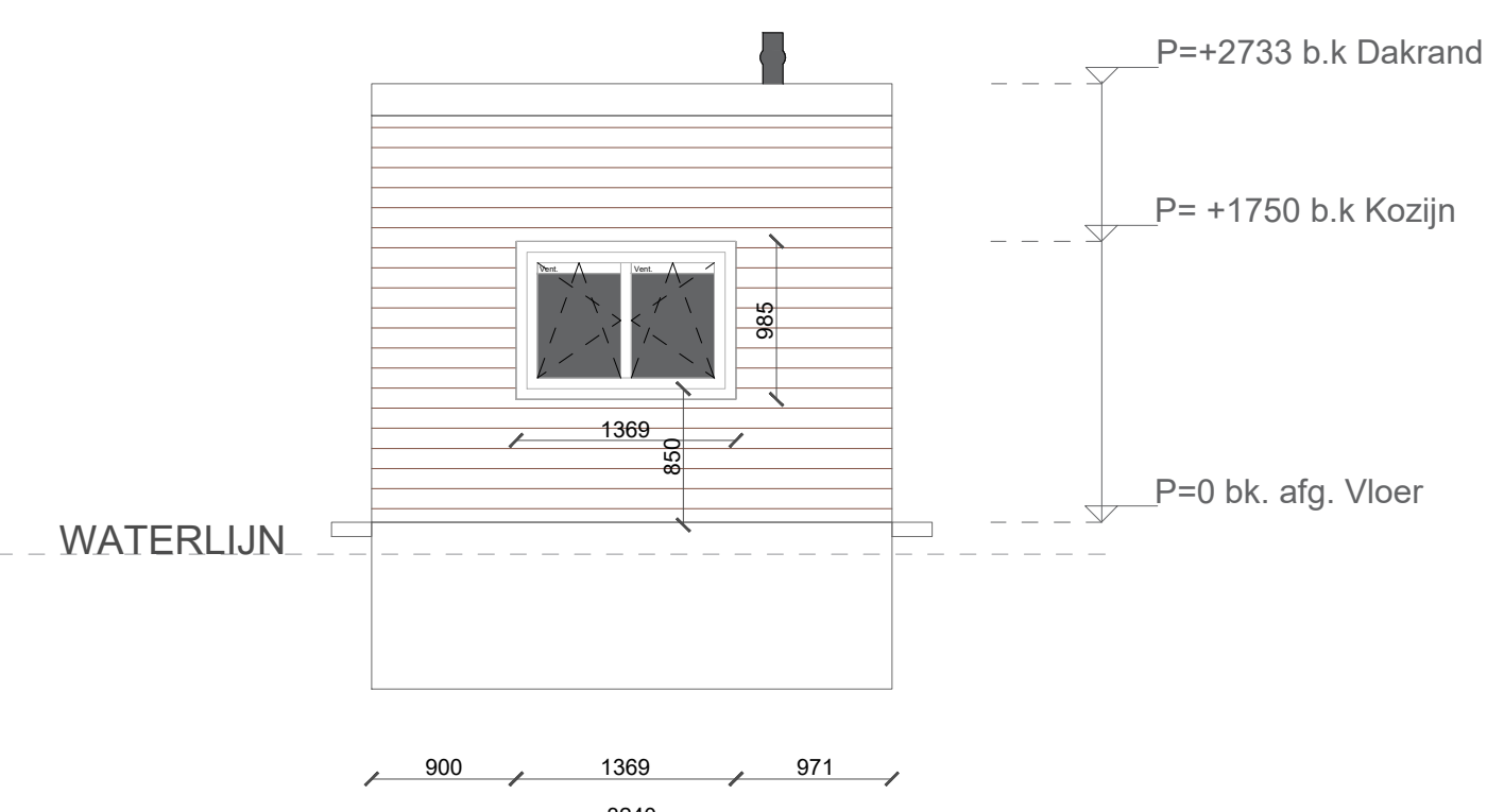
LINKERZIJGEVEL
