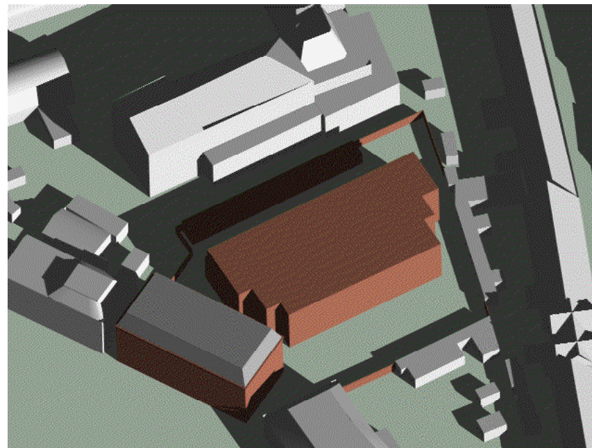
19 februari/21 oktober 1200 uur gebouw 90cm verschoven en 3 bouwlagen met setback
