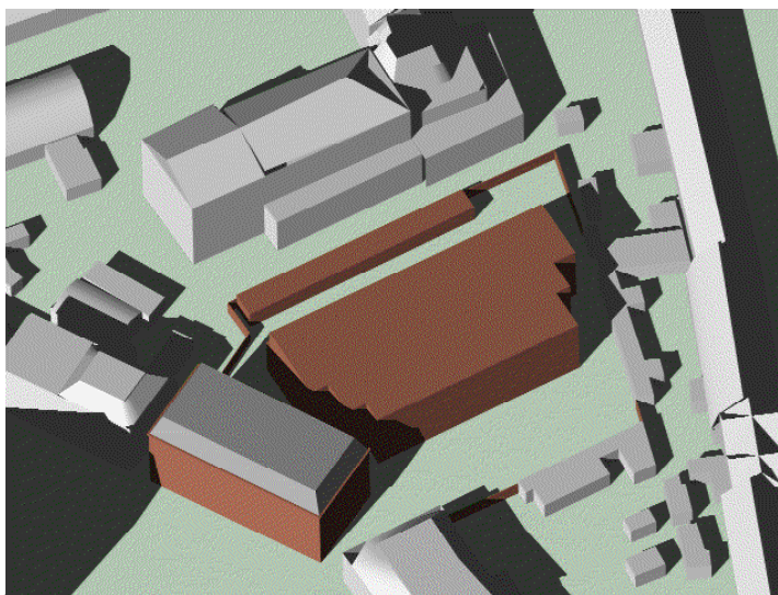
20 april/23 augustus 1700 uur gebouw 90cm verschoven en 3 bouwlagen met setback
