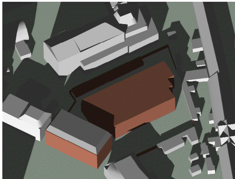
19 februari/21 oktober 1600 uur gebouw 90cm verschoven en 3 bouwlagen met setback
