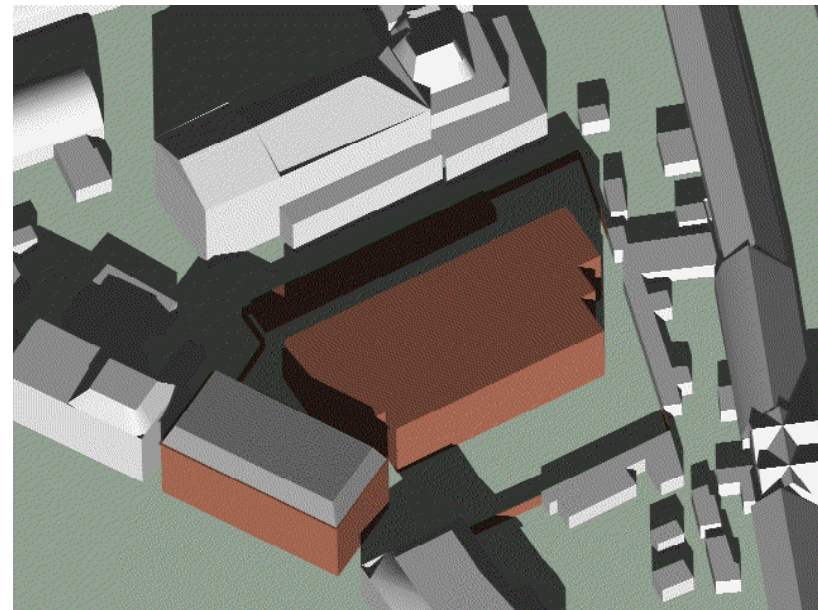
19 februari/21 oktober 1500 uur gebouw 90cm verschoven en 3 bouwlagen met setback
