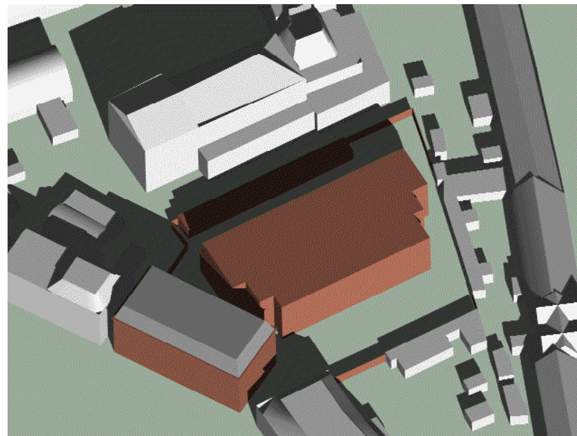
19 februari/21 oktober 1400 uur gebouw 90cm verschoven en 3 bouwlagen met setback
