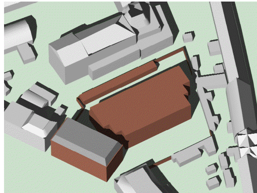
20 april/23 augustus 1600 uur gebouw 90cm verschoven en 3 bouwlagen met setback
