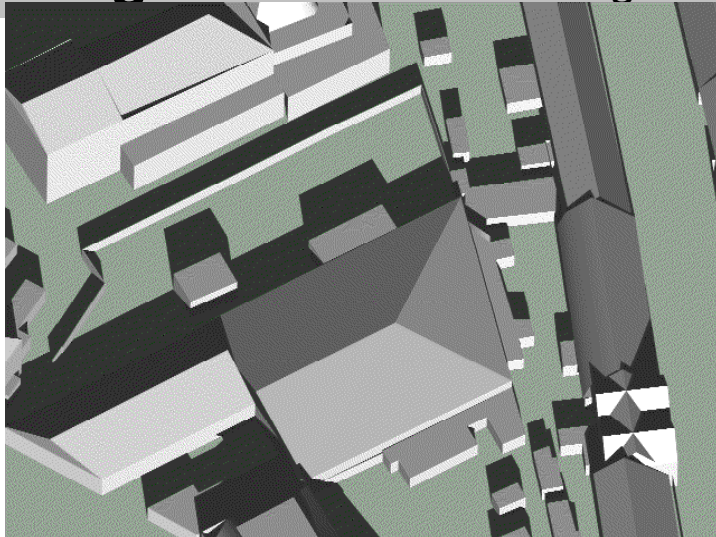
19 februari/21 oktober 1400 uur Huidige situatie
