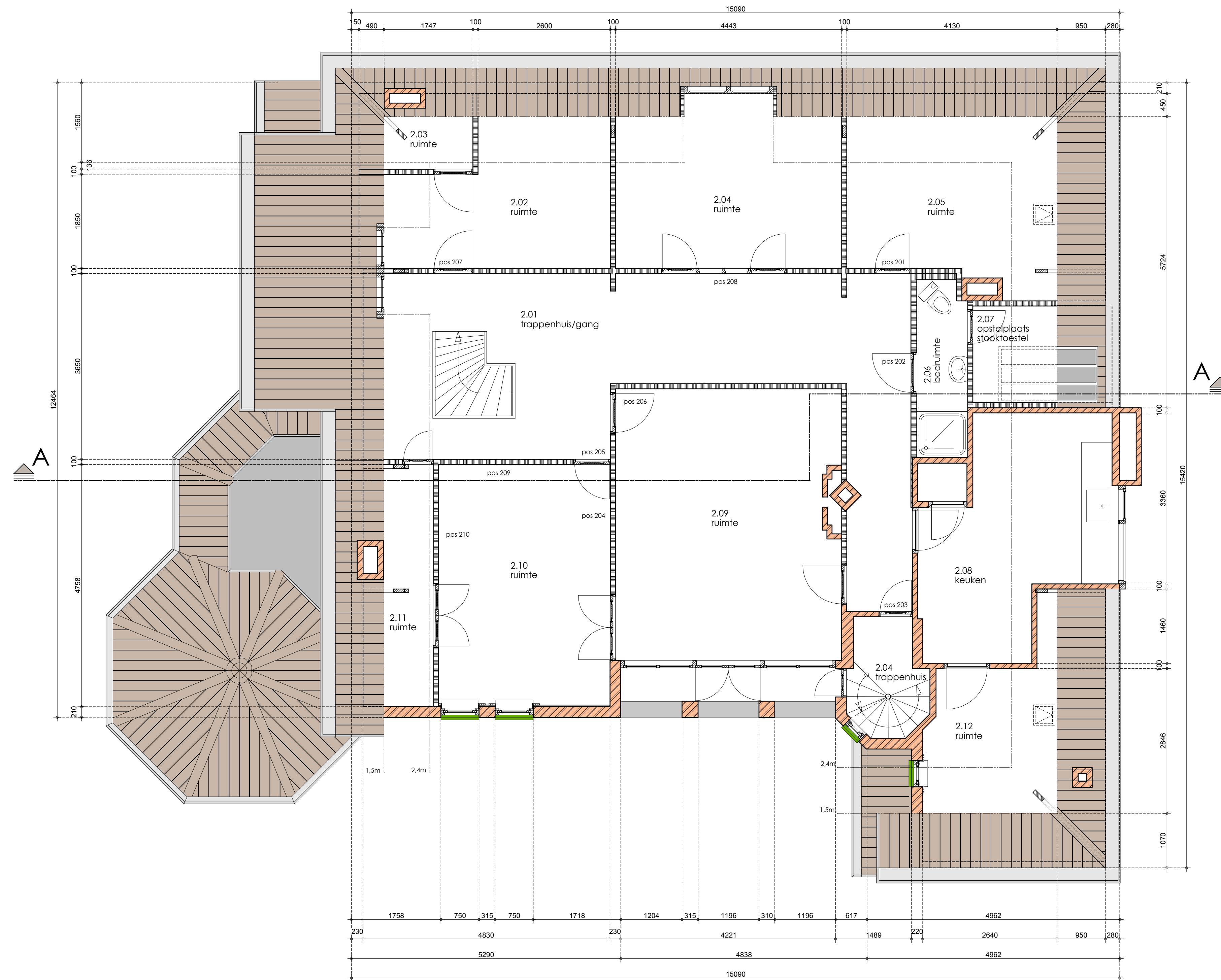
2e verdieping
