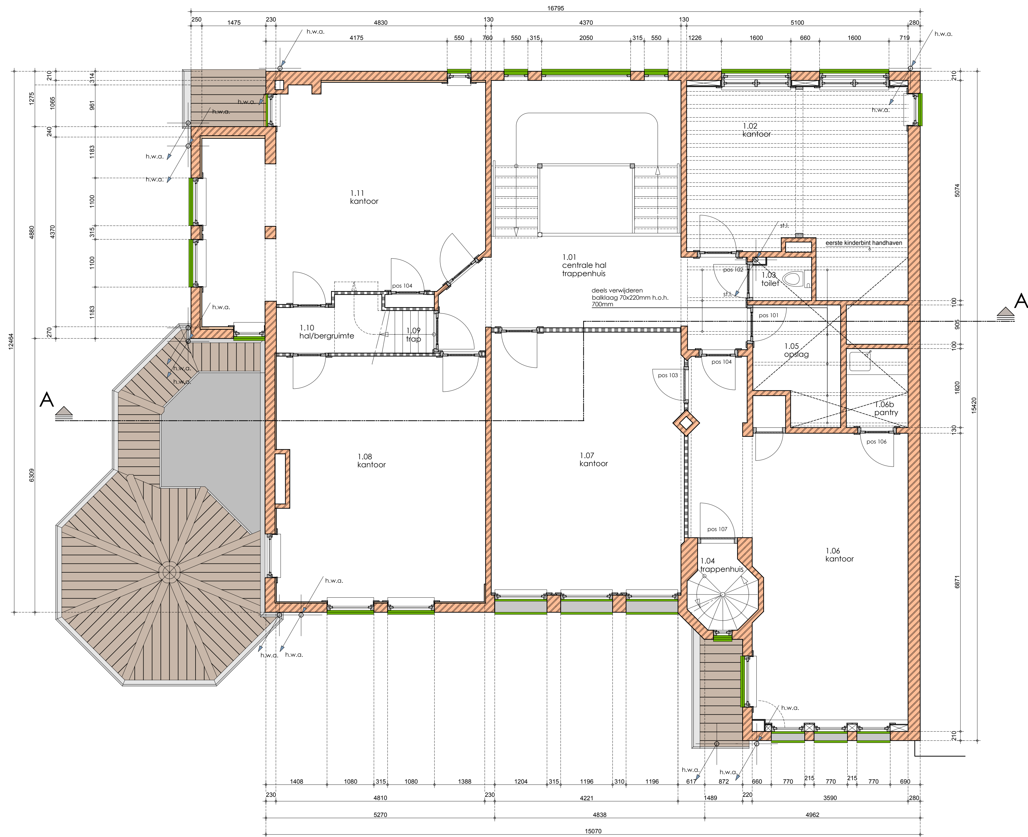
1e verdieping
