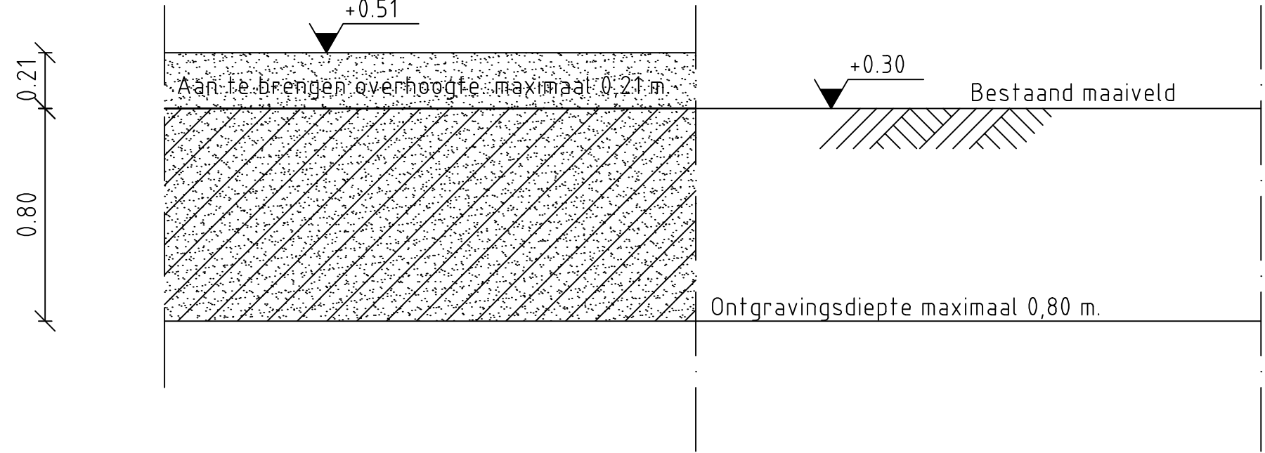
Doorsnede te ontgraven/op te hogen terrein Schaal 1:20
