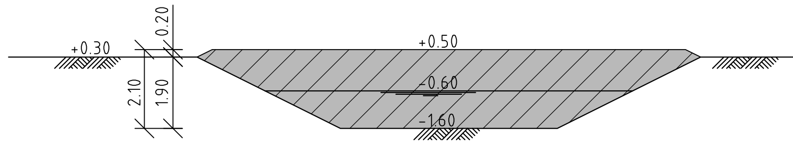
Doorsnede te dempen watergang Schaal 1:100
