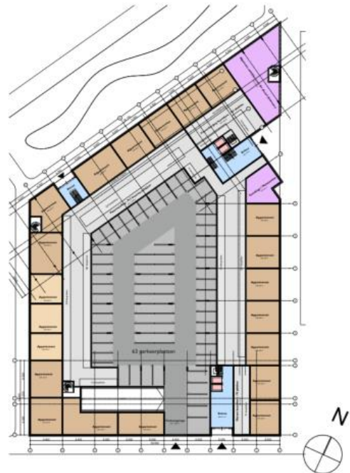
Begane grond
