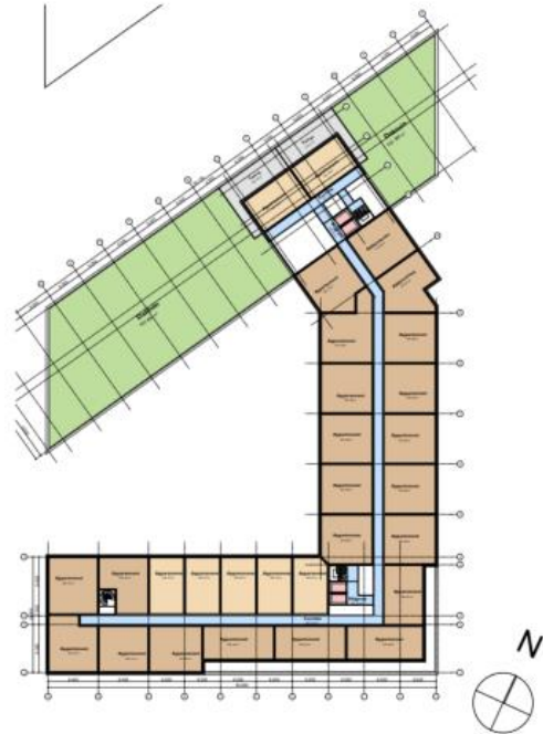
7e verdieping / Dak laagbouw
