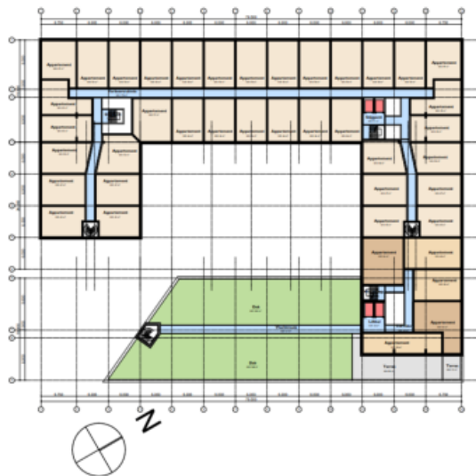
7e verdieping
