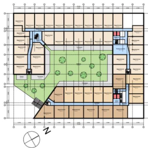
1e verdieping
