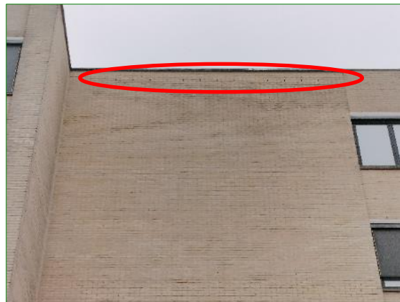
Rechts: Ook onder de rakrand zitten hier en daar rijen open stootvoegen.
