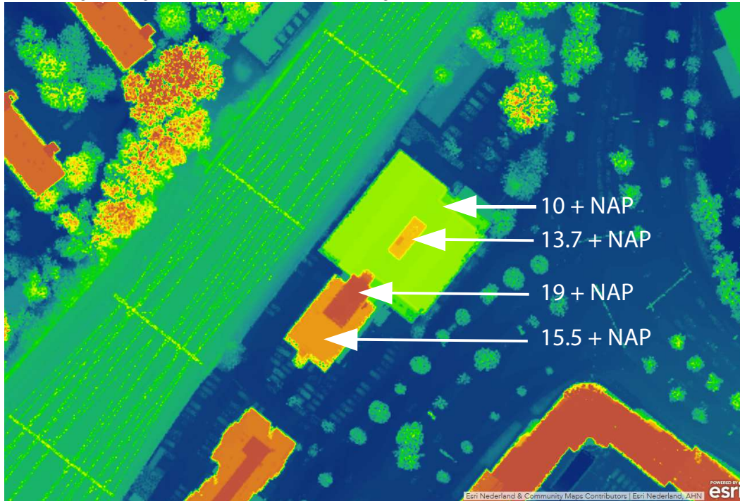
f2.2 Gebouwhoogten huidige situatie boven NAP (bron: AHN3 hoogtekkaart)
