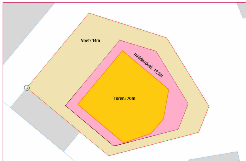
Figuur 3.2: Gebouwhoogte per deel
