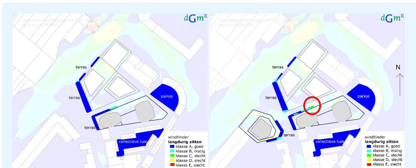
figuur 8: Links de nulsituatie. Rechts de nieuwe situatie met De Geus. Terrassen. Windhinder in windklassen A t/m E voor de activiteit 'langdurig zitten' met kwalificatie. Windklasse A betekent een goed windklimaat, windklasse B een matig windklimaat en windklassen C, D en E een slecht windklimaat.
