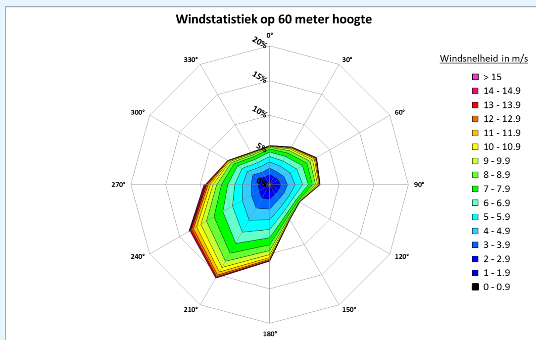
figuur 3: Windstatistiek Leiden
