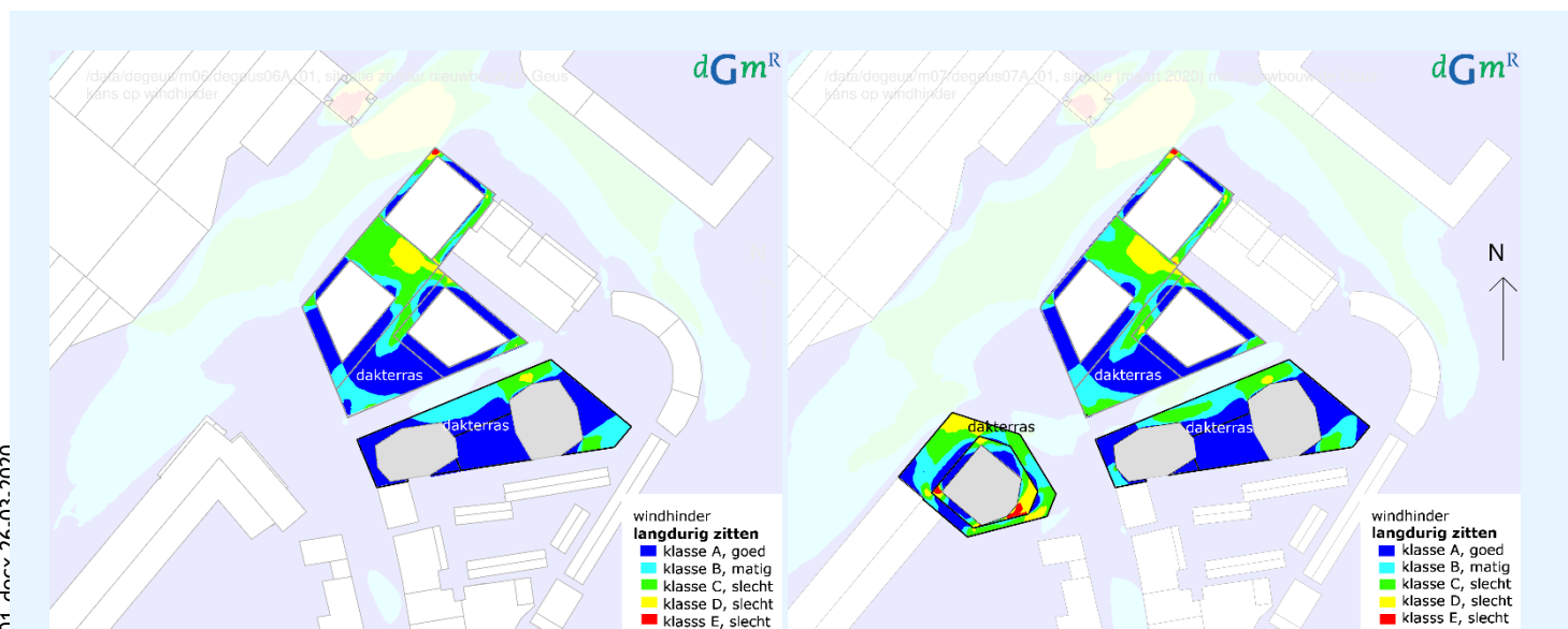
figuur 9: Links de nulsituatie. Rechts de nieuwe situatie met De Geus. Dakterrassen. Windhinder in windklassen A t/m E voor de activiteit 'langdurig zitten' met kwalificatie. Windklasse A betekent een goed windklimaat, windklasse B een matig windklimaat en windklassen C, D en E een slecht windklimaat.
