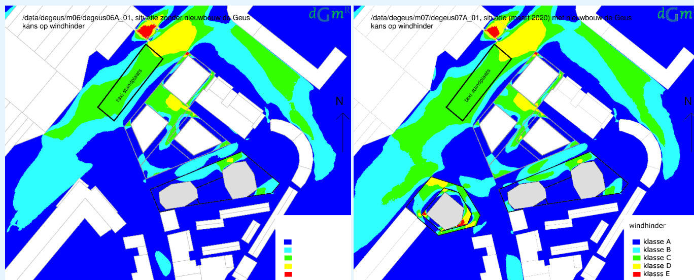
figuur 5: Links de nulsituatie. Rechts de nieuwe situatie met De Geus.
