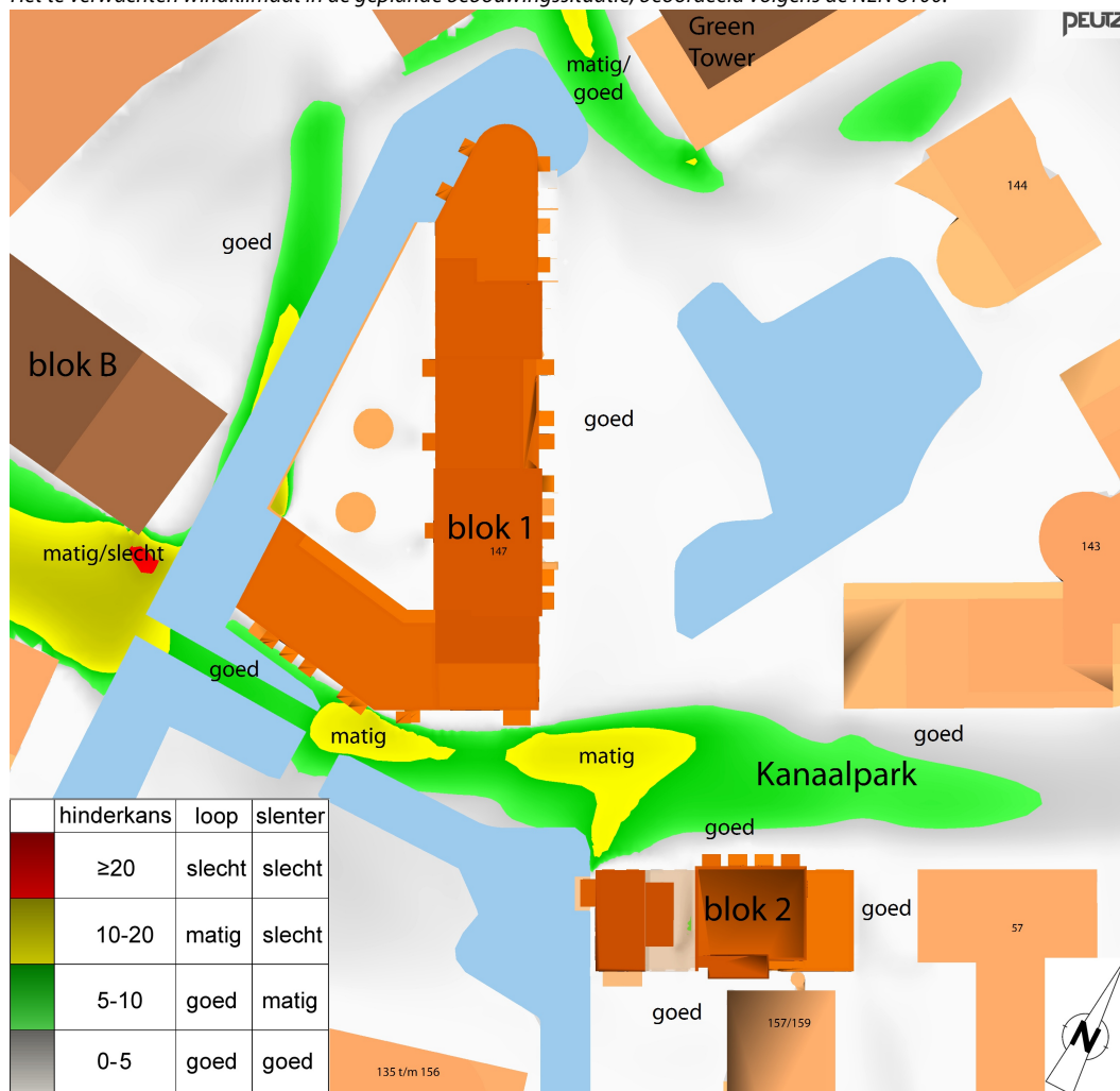
f3.2 Het te verwachten windklimaat in de geplande bebouwingssituatie, beoordeeld volgens de NEN 8100.
