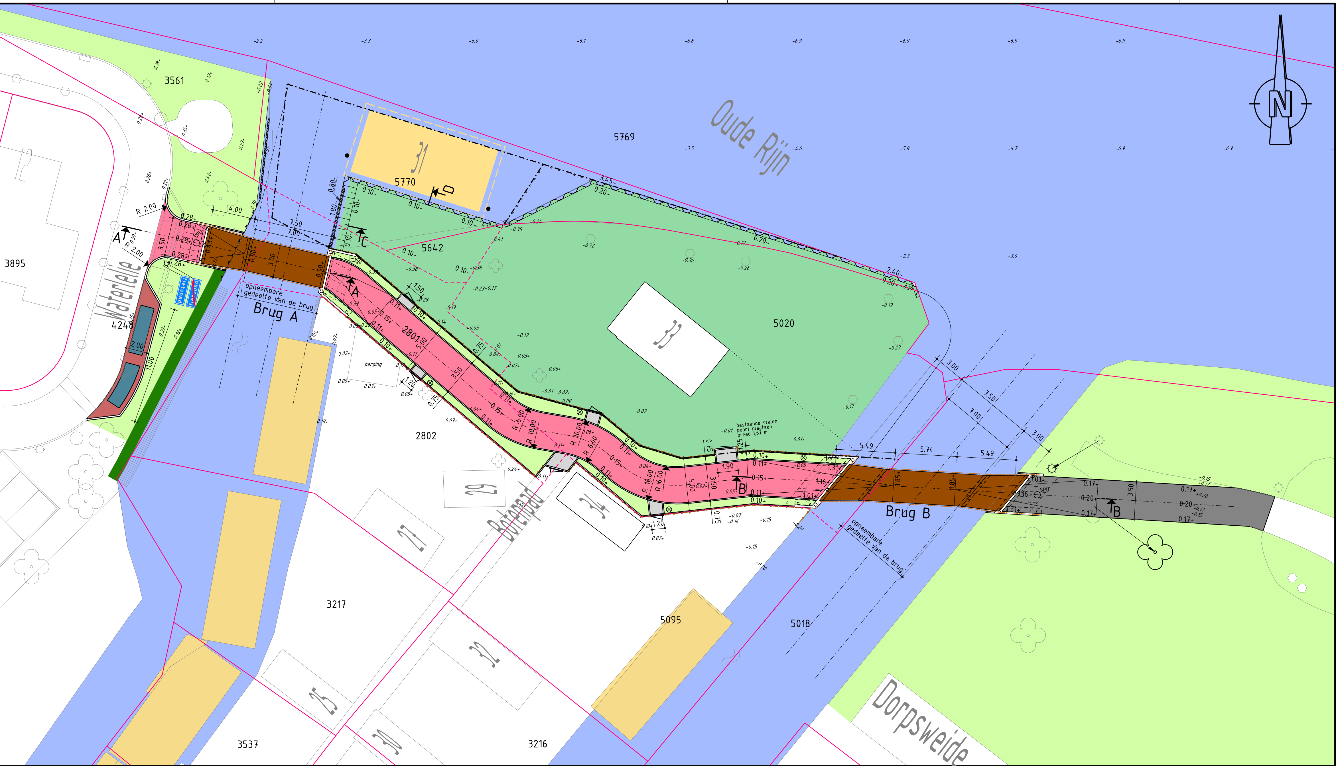
Situatie Schaal 1:200
