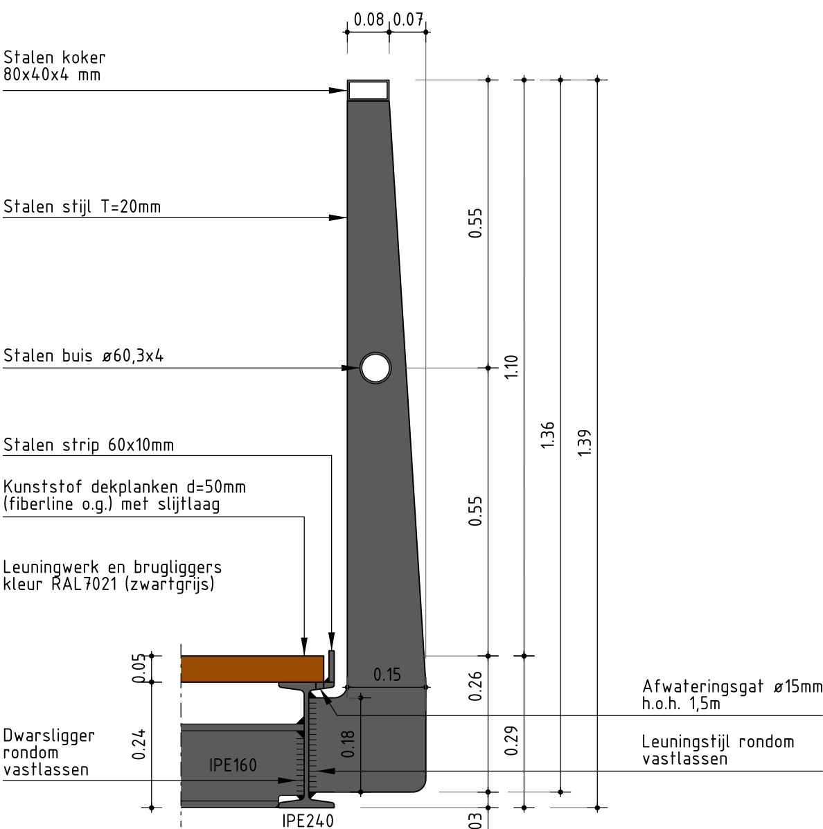
Detail leuning Schaal 1:20
