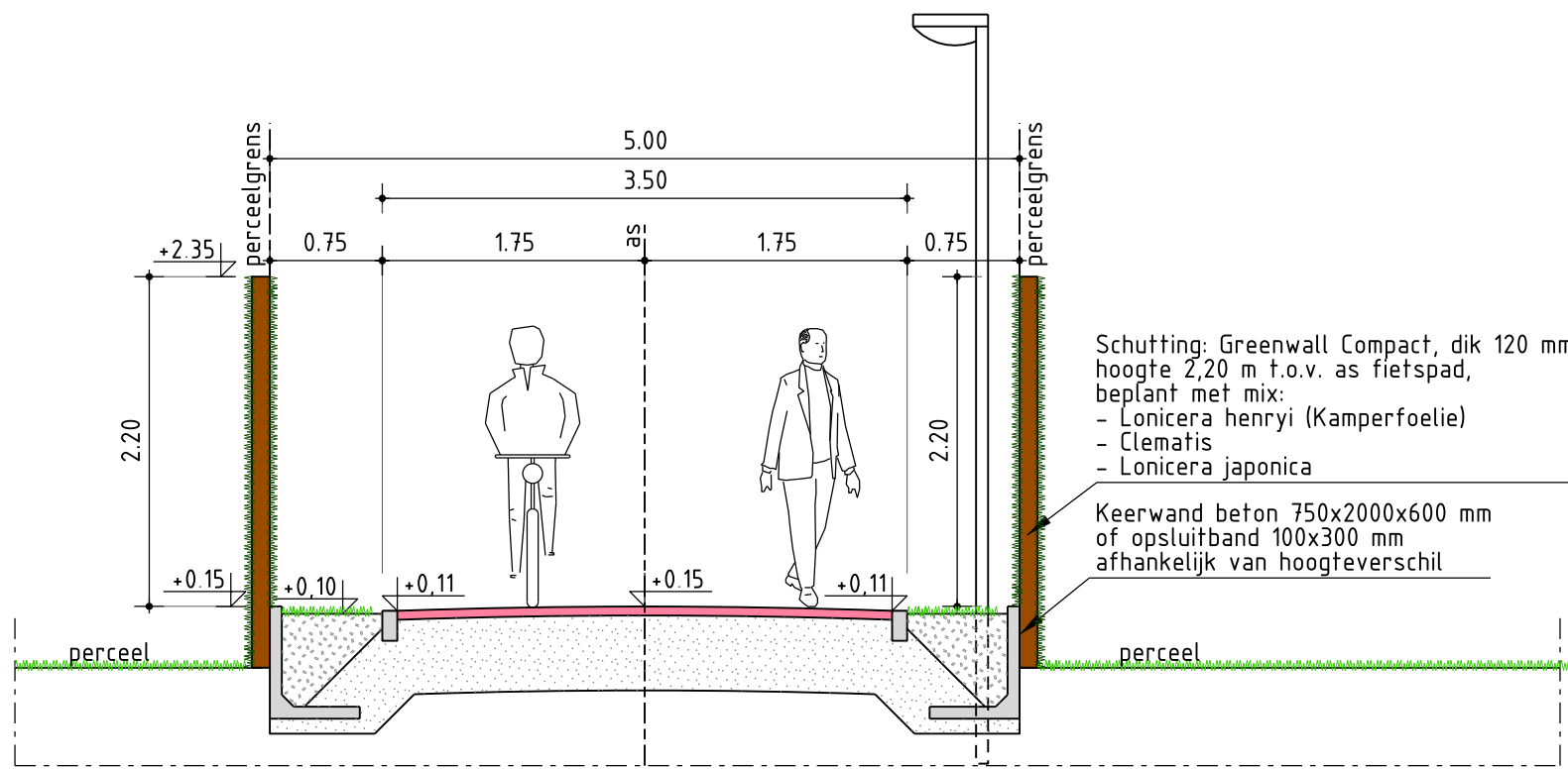
Principeddoorsnede fietspad Schaal 1:50
