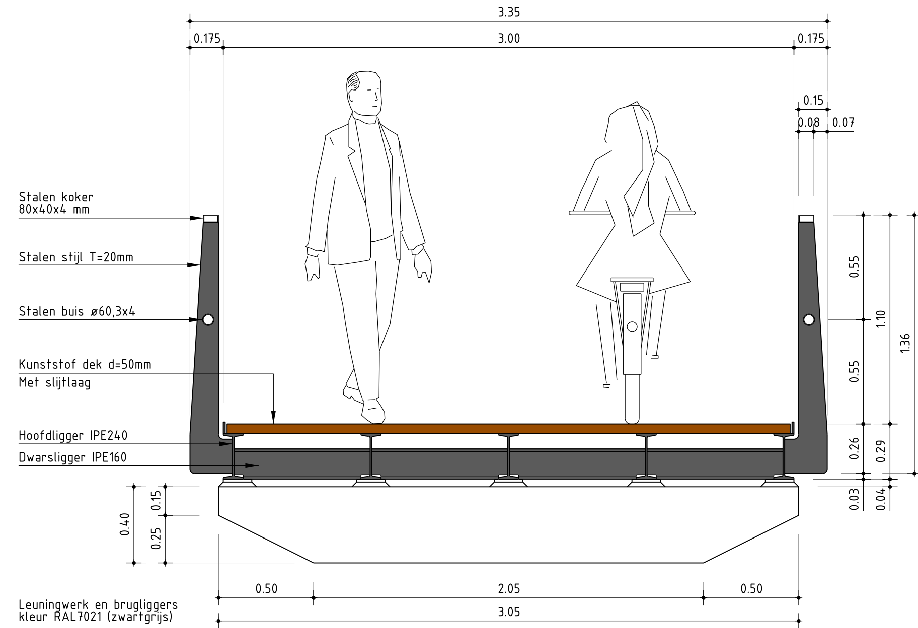
Principeddoorsnede brug Schaal 1:20
