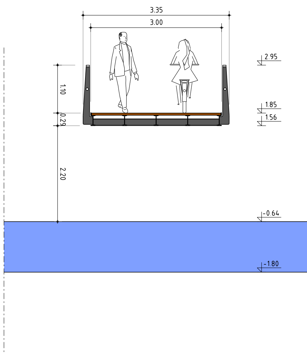
Dwarsdoorsnede brug B Schaal 1:50
