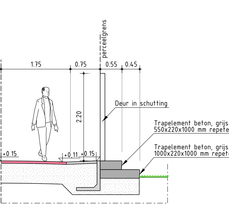
Principeddoorsnede trap Schaal 1:50
