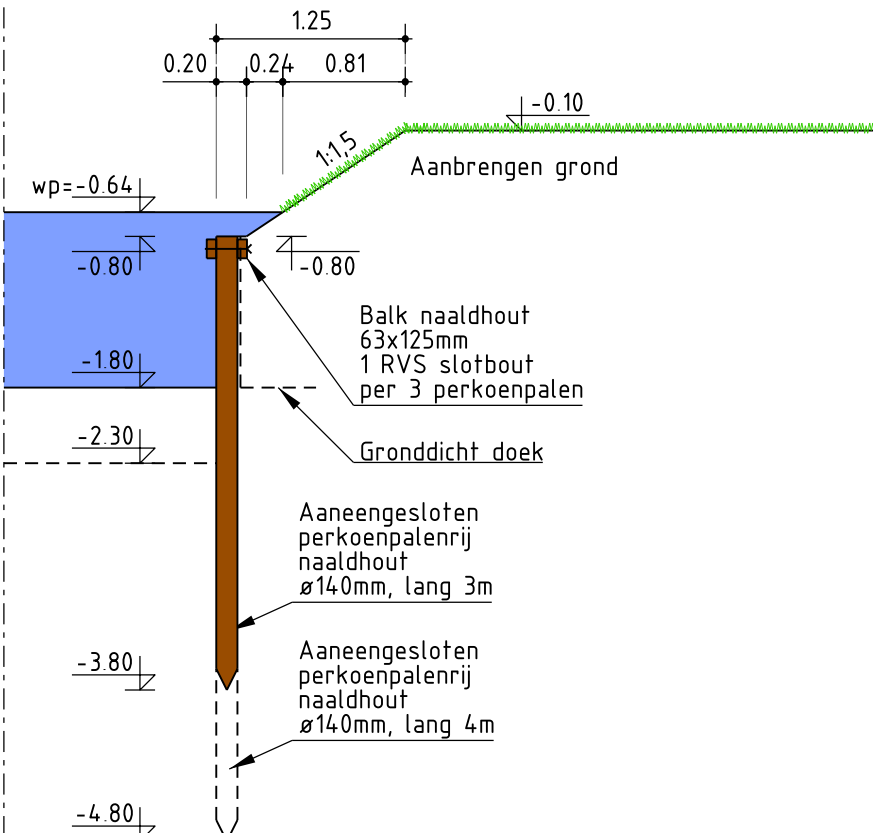
Doorsnede C Schaal 1:50
