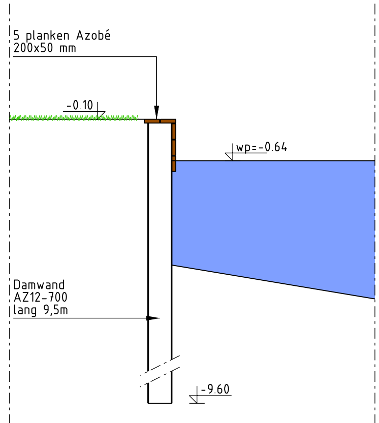
Doorsnede D Schaal 1:50
