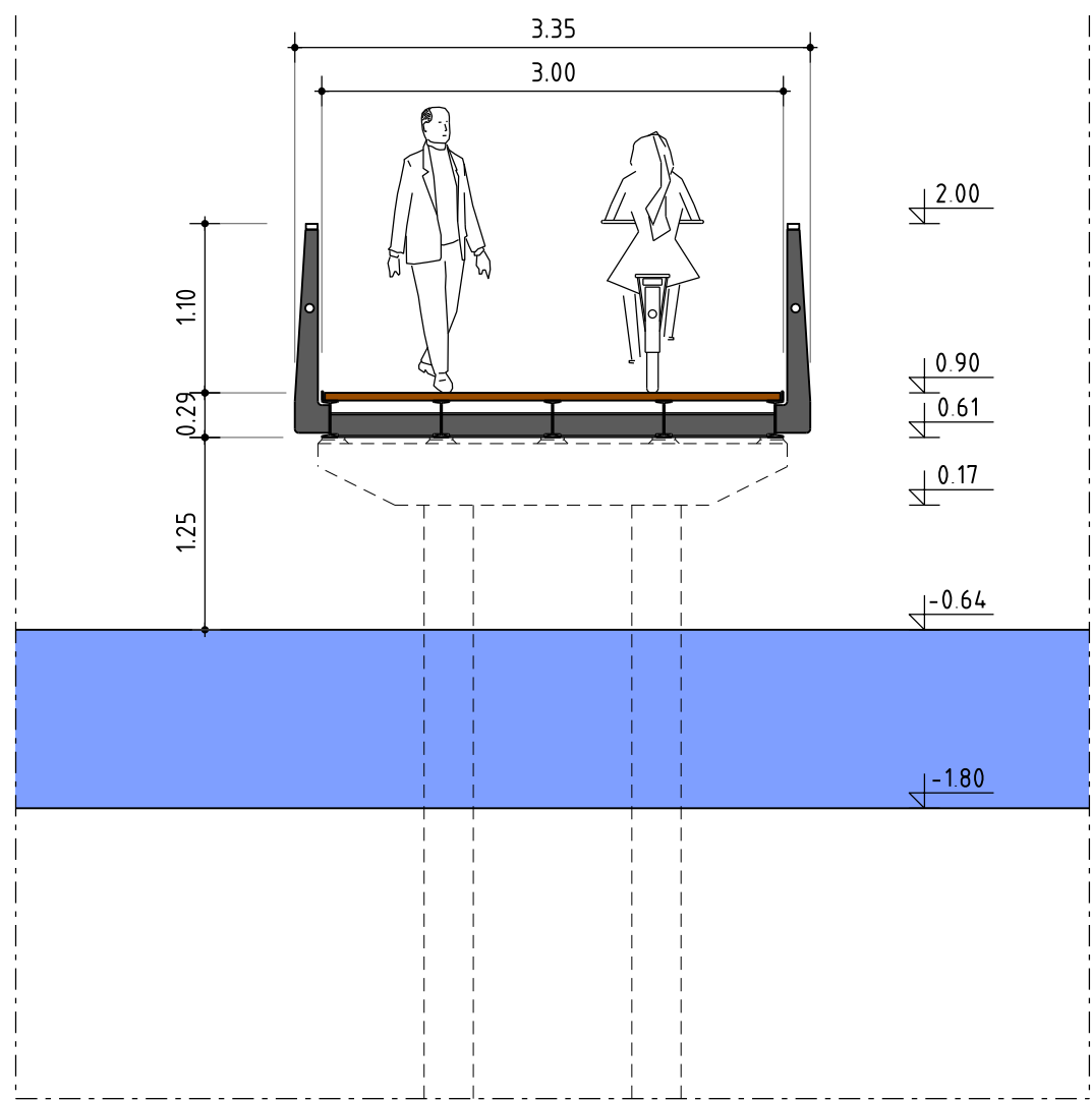
Dwarsdoorsnede brug A Schaal 1:50
