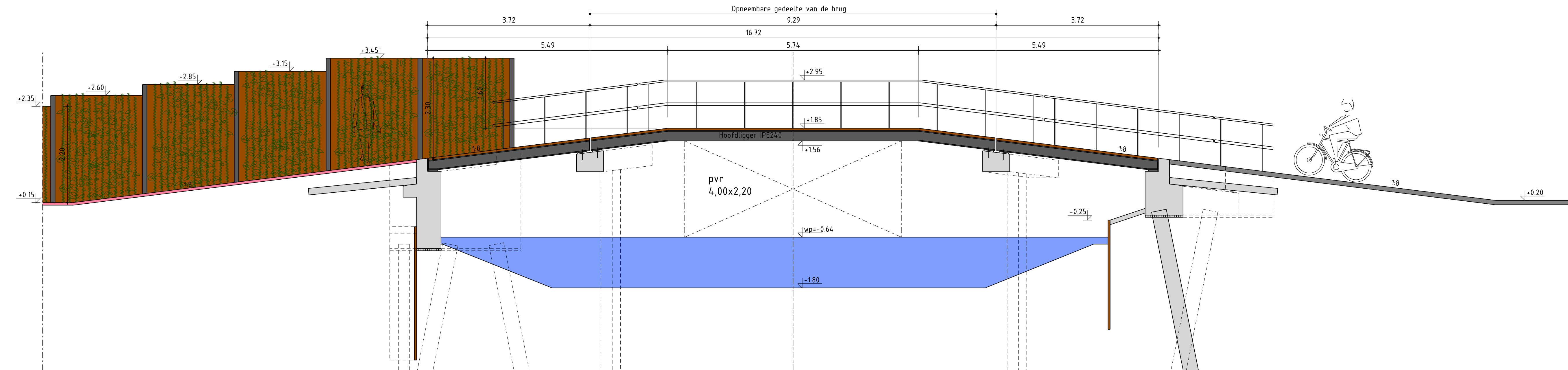
Doorsnede B-B Schaal 1:50
