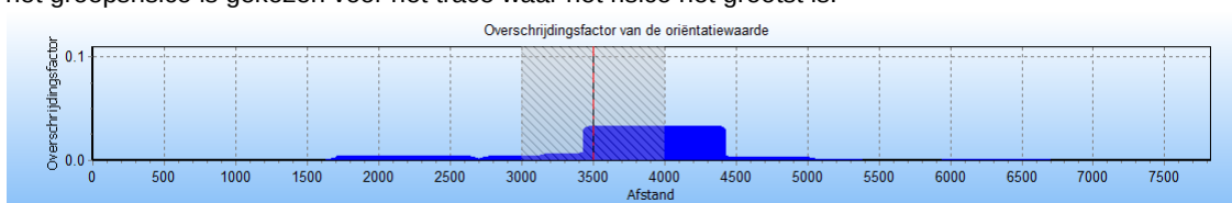
Figuur 5 Overschrijding van het groepsrisico als functie van de stationing van W-535-01 in de huidige situatie.
