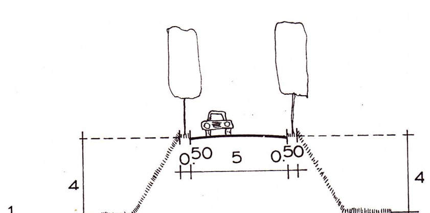
WEGPROFIELEN SCHAAAL 1:200
