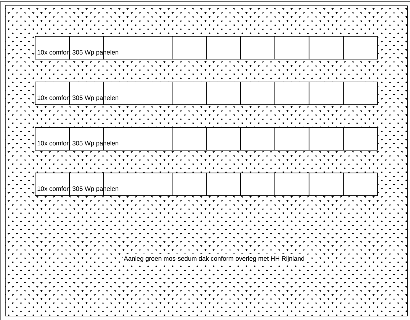
Dakvloer 7000+
