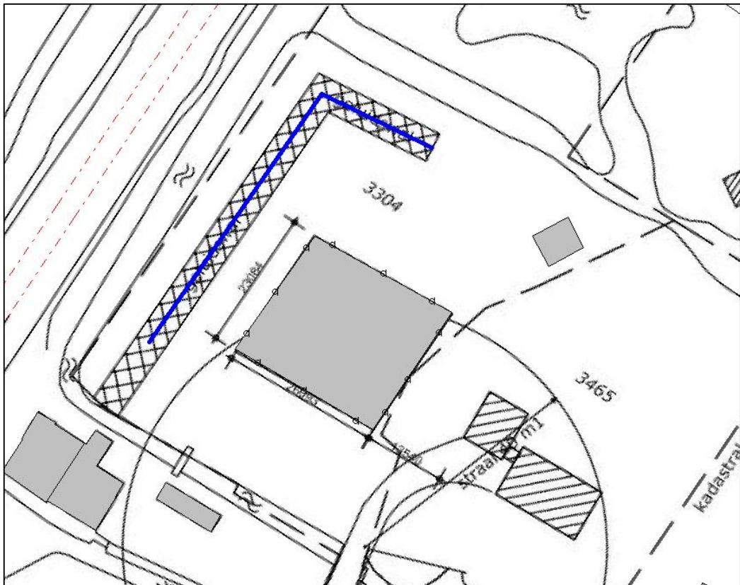
Figuur 4.1: Situering geluidwal (blauwe lijn) met een hoogte van 4 meter boven plaatselijk maaiveld
