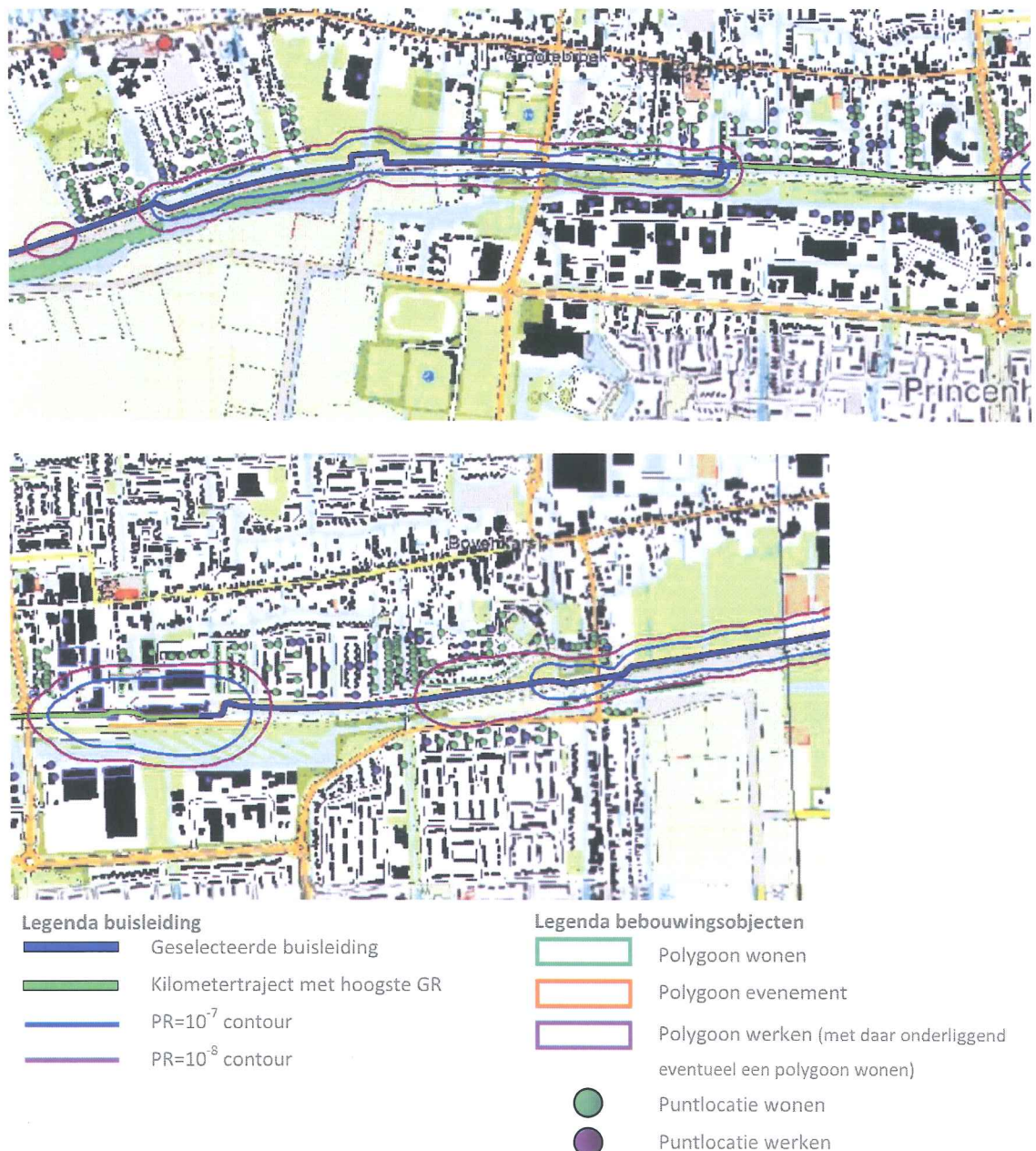
Figuur 5.1: Ingevoerde omgevingsobjecten in CAROLA en PR-contouren en hoogste GR-tracé leiding W-573-05
