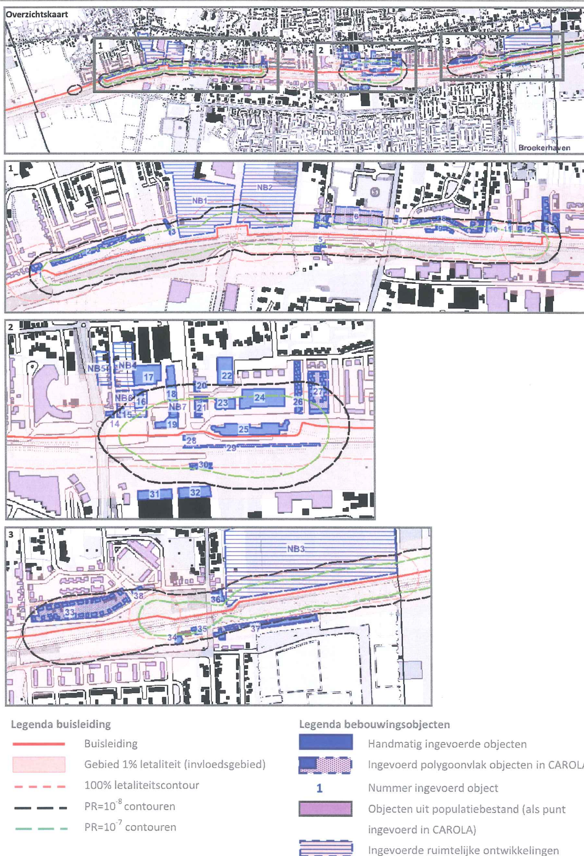
Figuur 4.2: Ingevoerde omgevingsobjecten en ligging 1% en 100% letaliteitscontouren en PR-contouren
