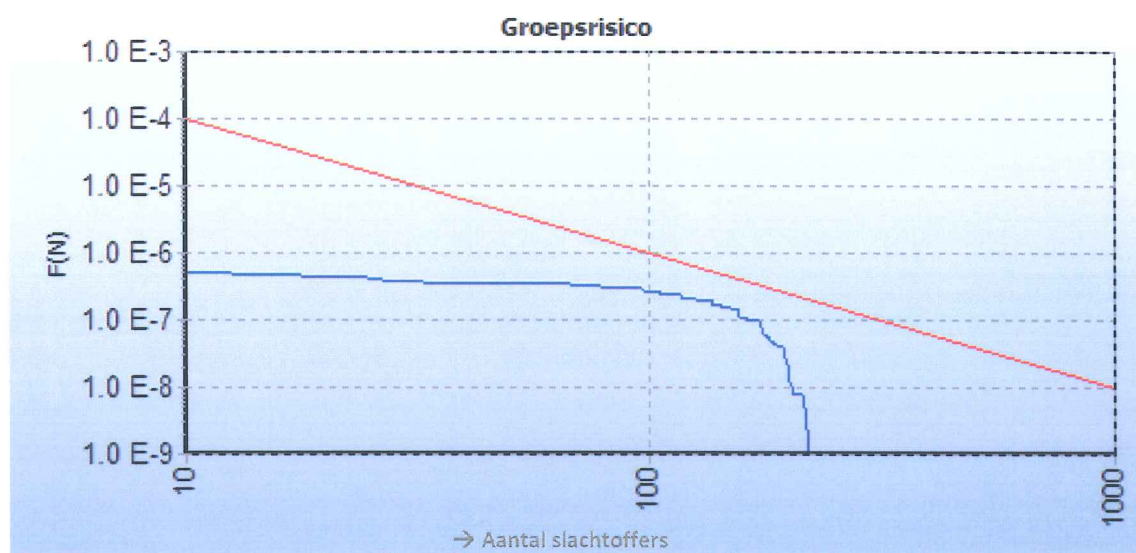
Figuur 5.3 FN curve voor W-573-05 van N.V. Nederlandse Gasunie voor de kilometer tussen stationing 4110.00 en stationing 5110.00. (bestaande situatie en toekomstige situatie)
