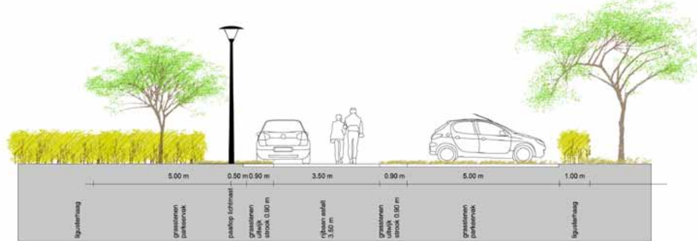
Doorsnede D-D'
