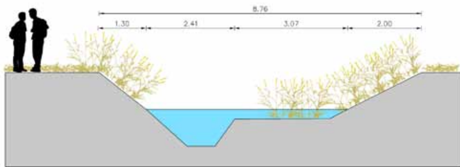
Doorsnede A-A'
