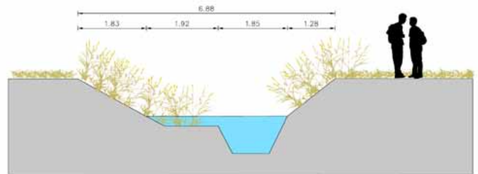
Doorsnede B-B'
