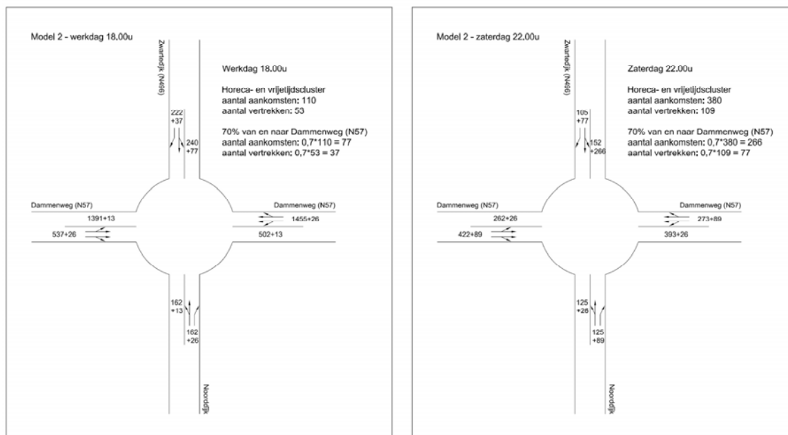
Fig. 9. Verkeersintensiteiten (gedurende één uur) 2020 na realisatie voorgenomen activiteit
