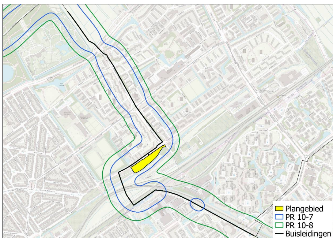
Figuur 3. PR-contouren aardgasleiding W-514-16
