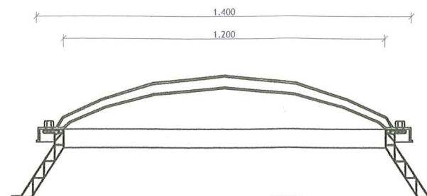
BIK polycarbonaat dubbelwandige lichtkoepel Afm.: 1200 x 1200 mm (dagmaat) Aantal: 1 stk
