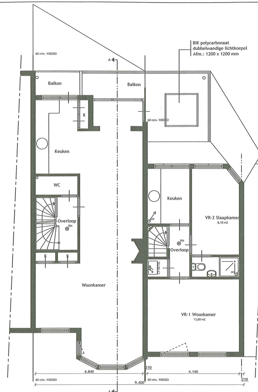
PLATTEGROND 1E VERDIEPING
