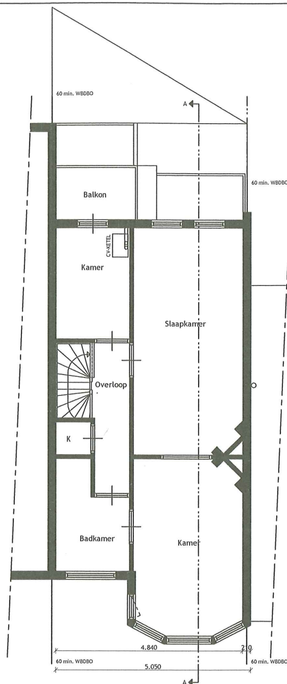
PLATTEGROND 2E VERDIEPING (ongewijzigd)
