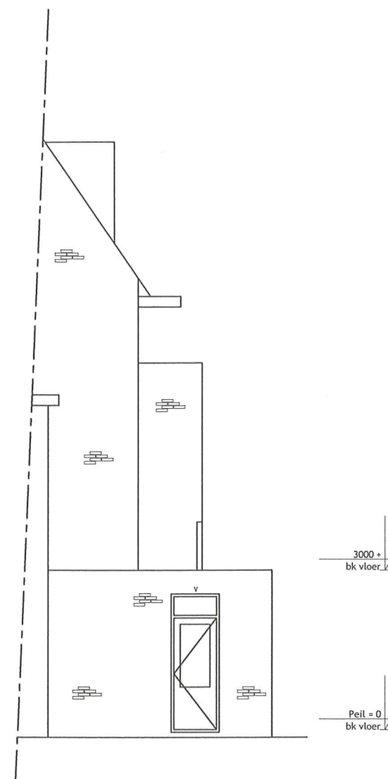
ZIJGEVEL T.P.V. SLAAPKAMER (NR. 74)
