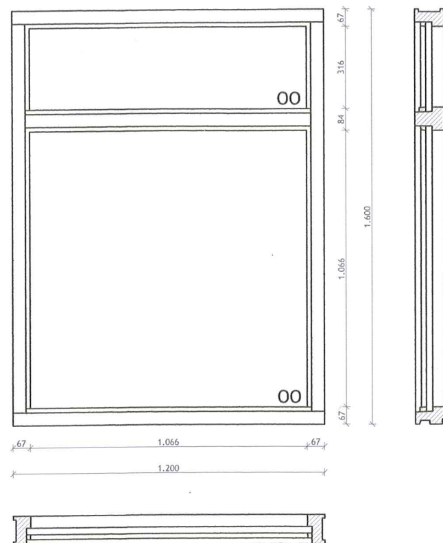
H-01 Meranti houten gevelkozijn Aantal: 1 stk
