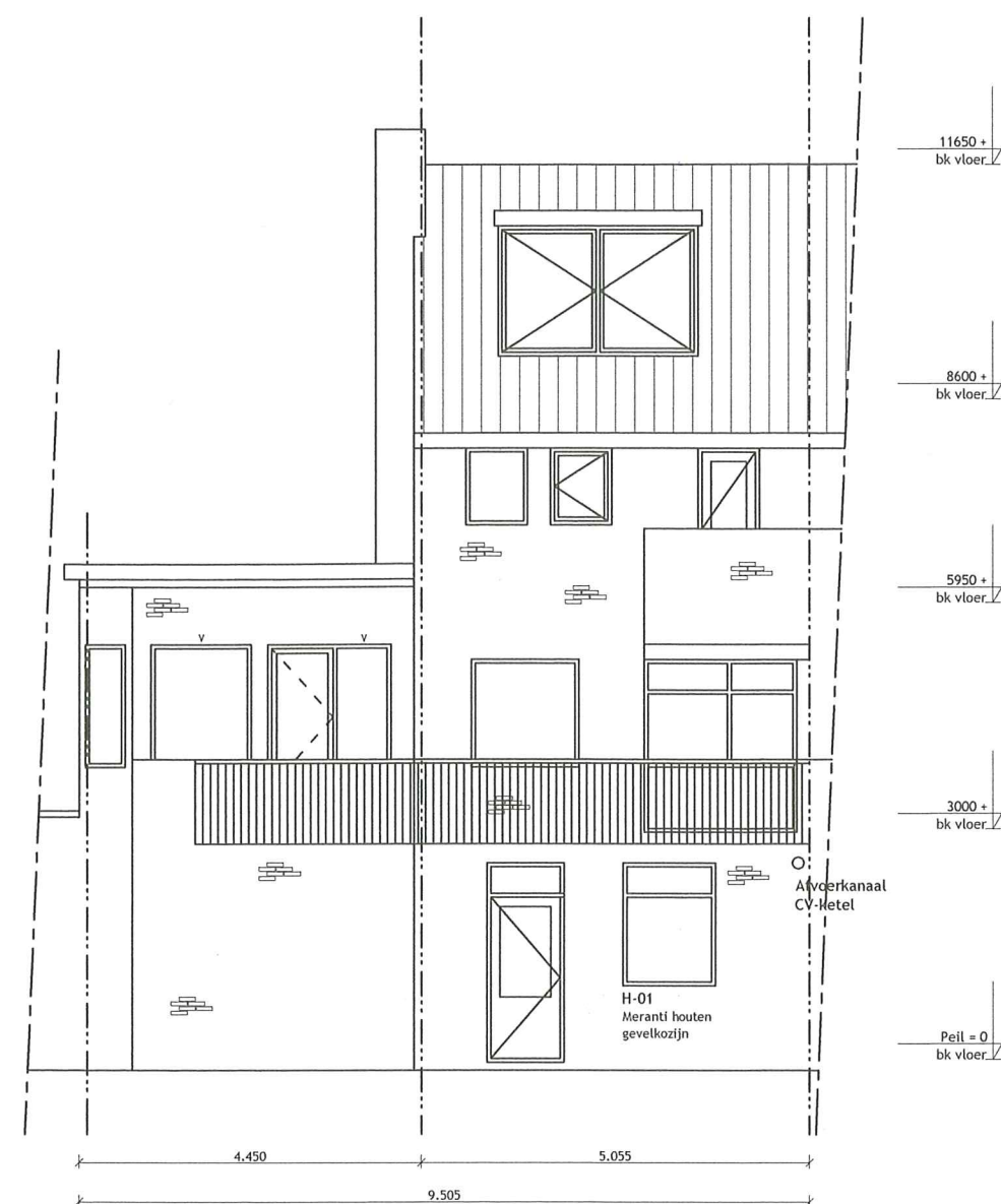
ACHTERGEVEL
