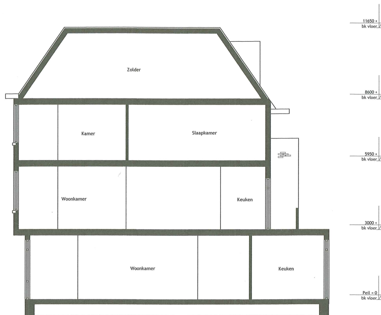
DOORSNEDE A-A
