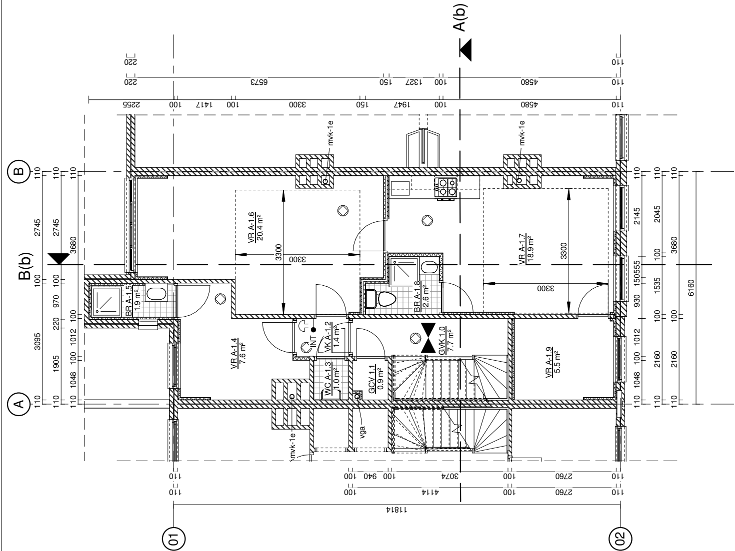
1e verdieping - bestaand
