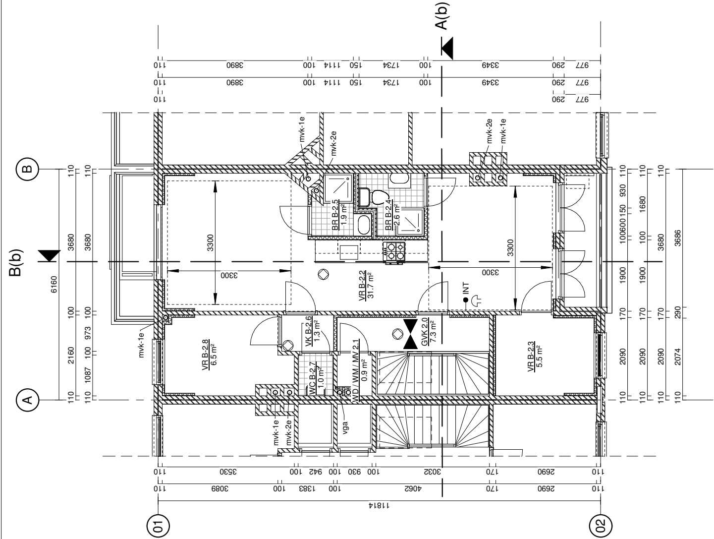
2e verdieping - bestaand
