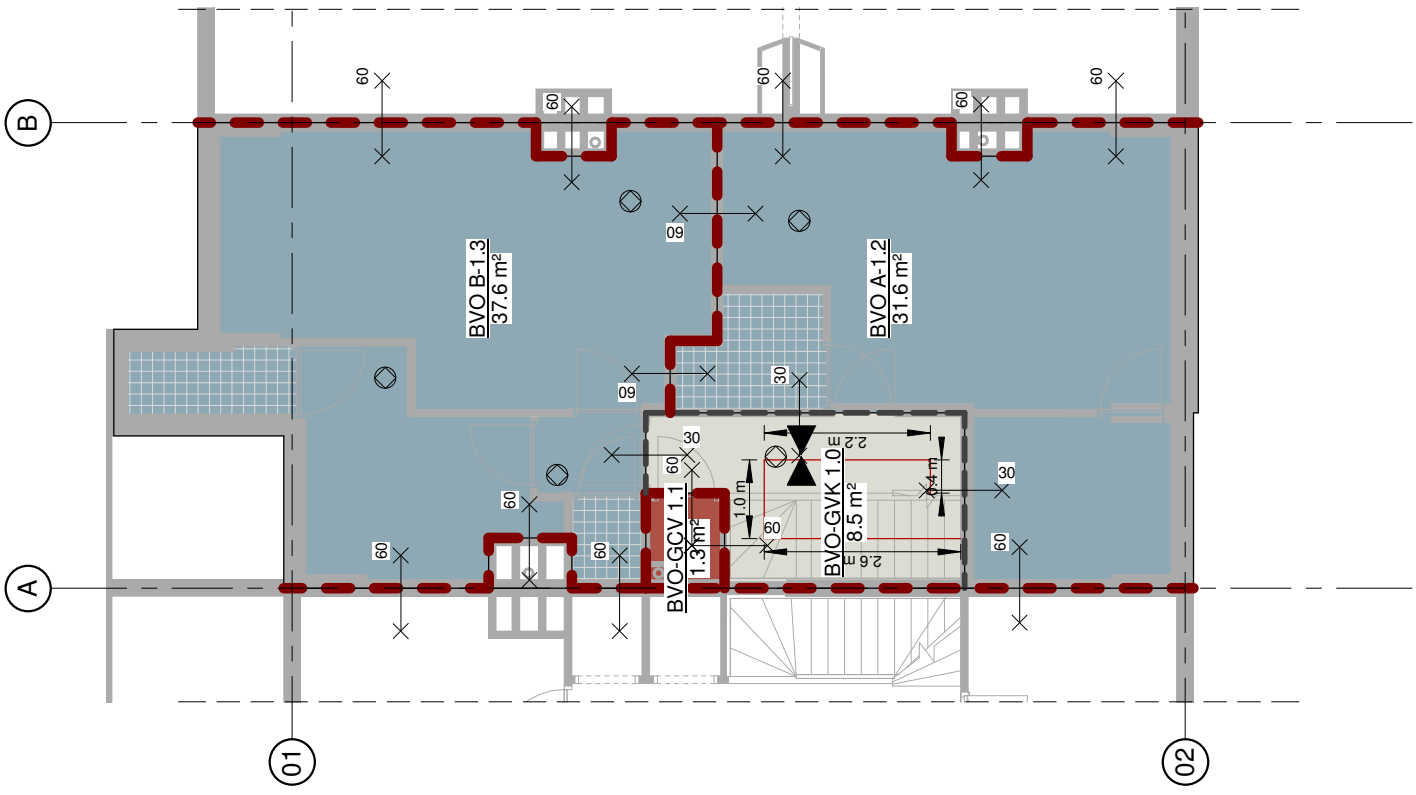
BVO - 1e verdieping
