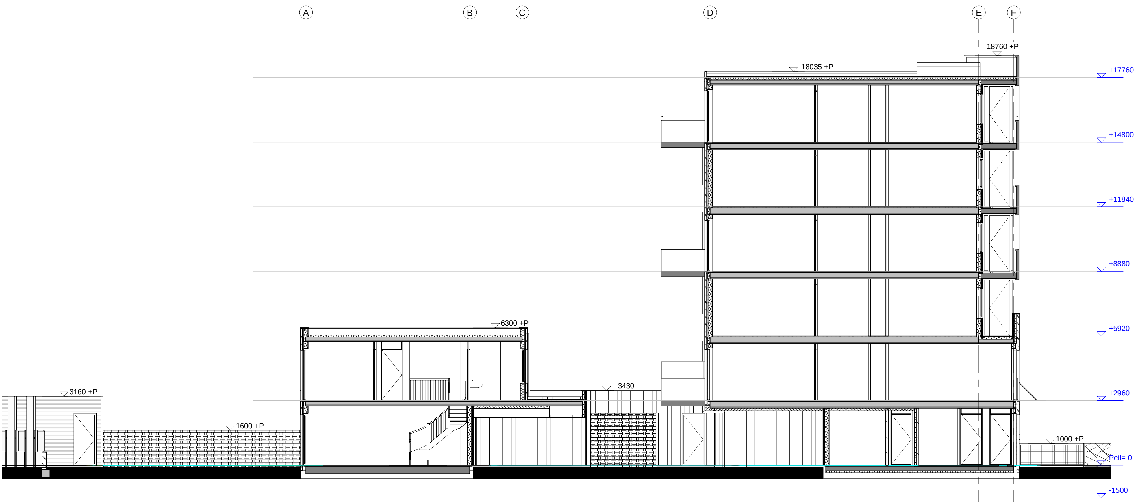
Doorsnede A-A
