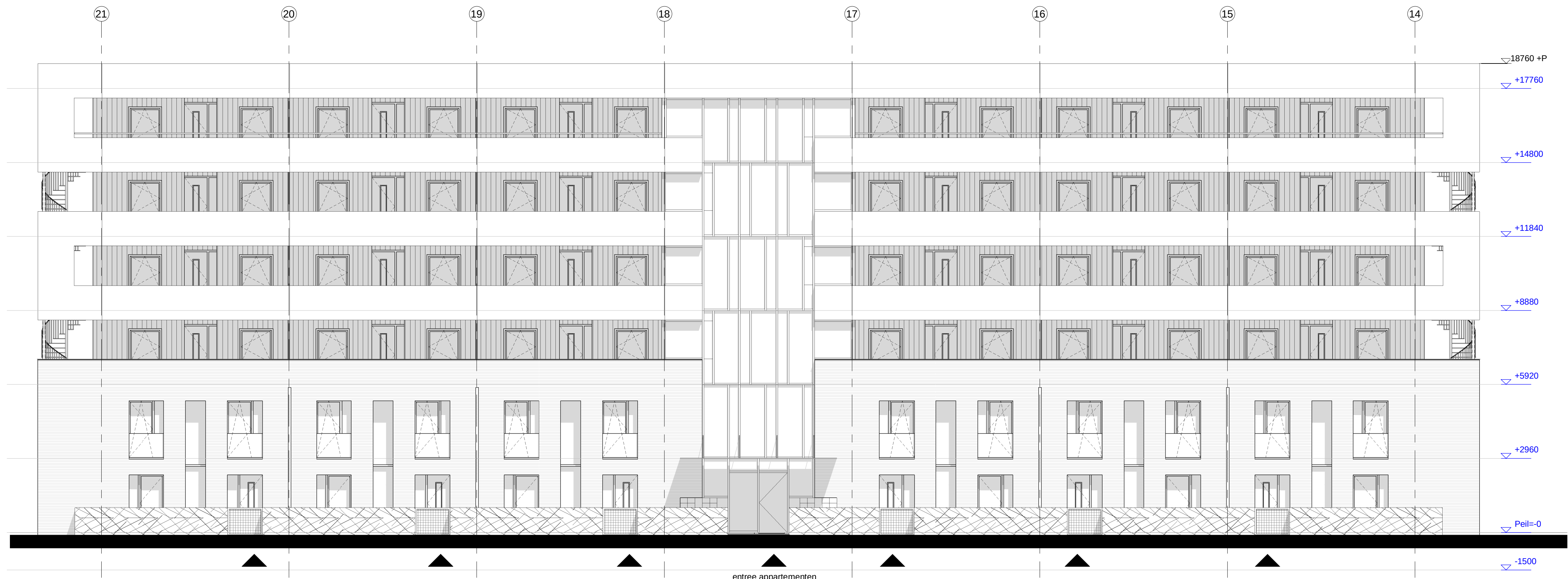
Straatgevel Meppelweg
