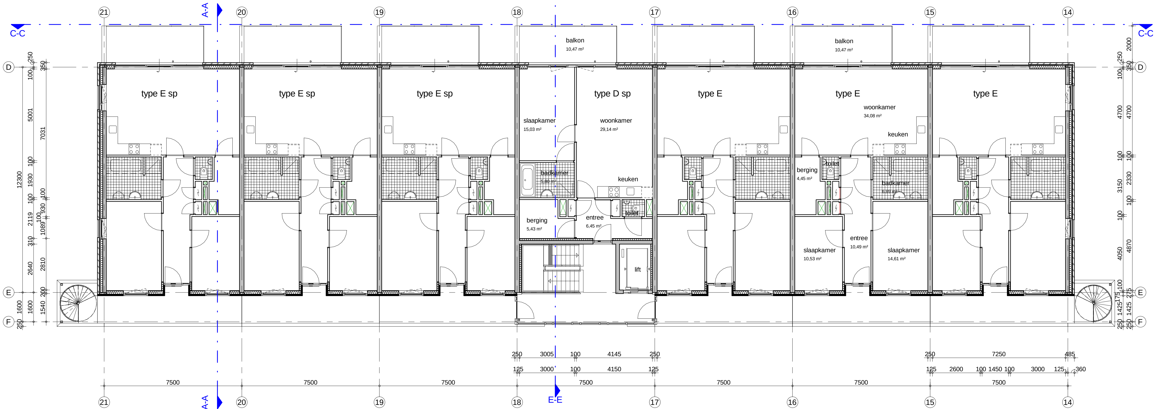
4e Verdieping
