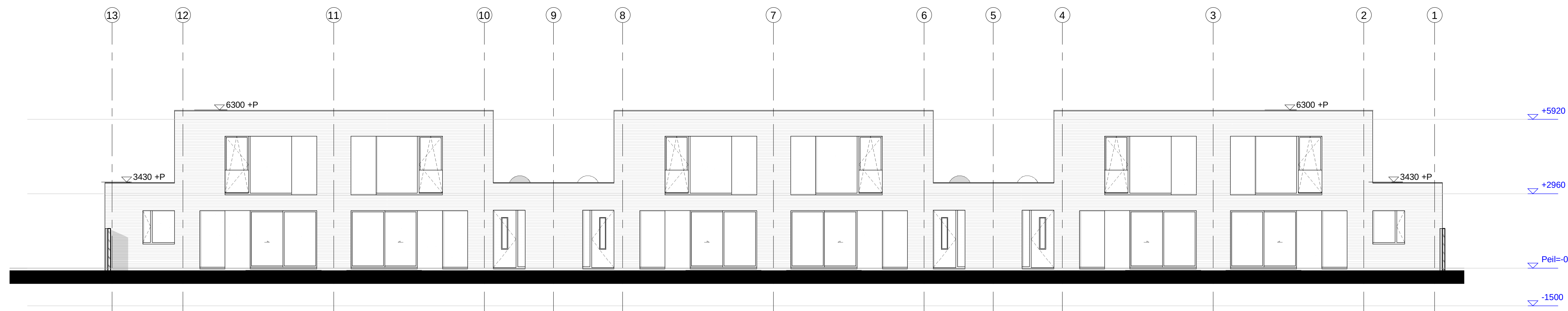
Voorgevel grond gebonden woningen, doorsnede D-D
