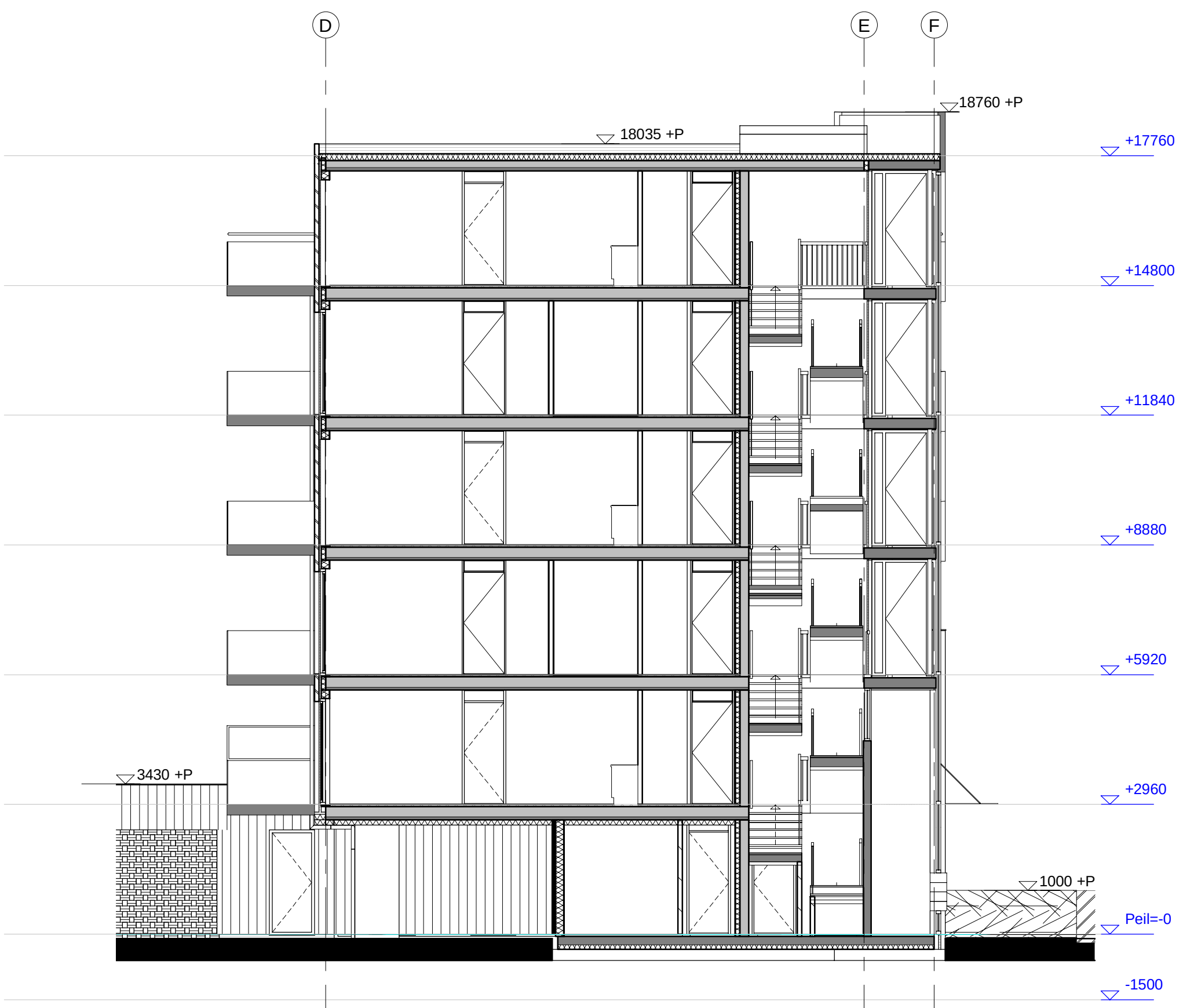
Fragment doorsnede E-E
