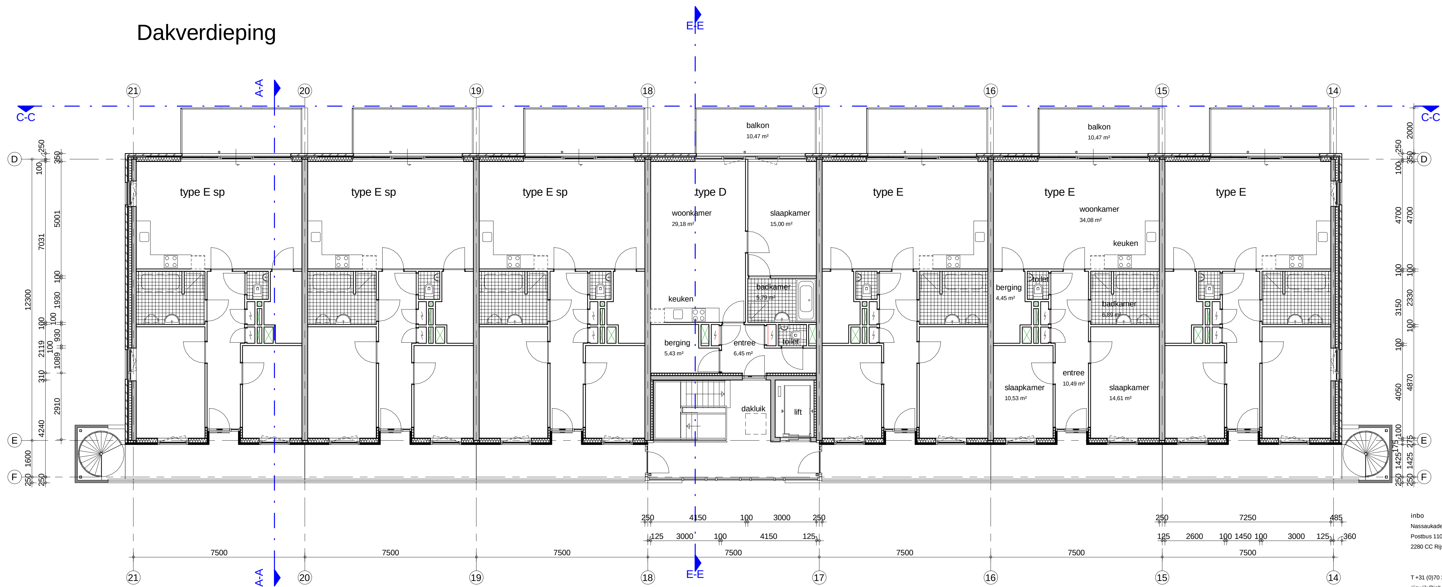
5e Verdieping
