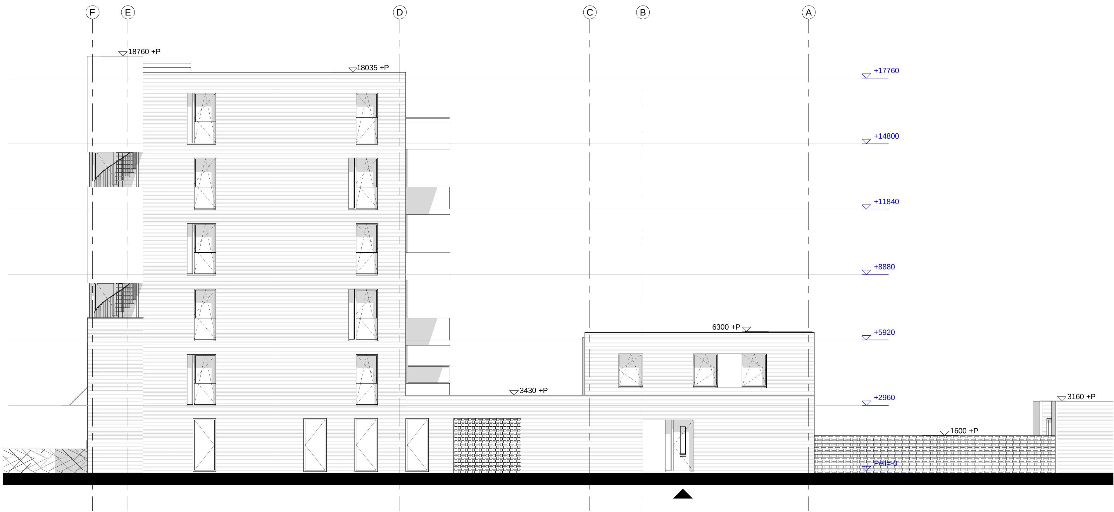
Straat aanzicht Gietenstraat
