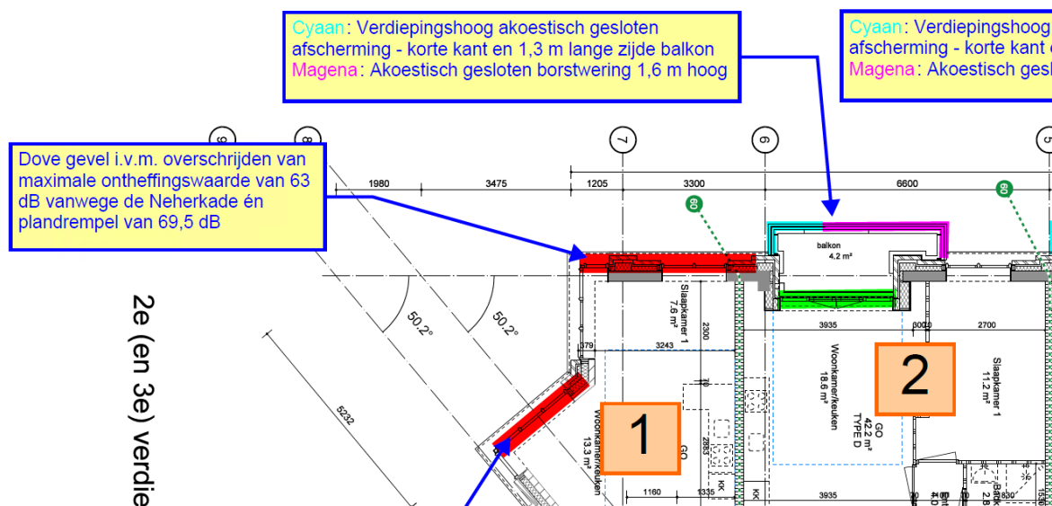
Figuur 3: Balkonscherm bij appartement met nr. 2 meer in detail
