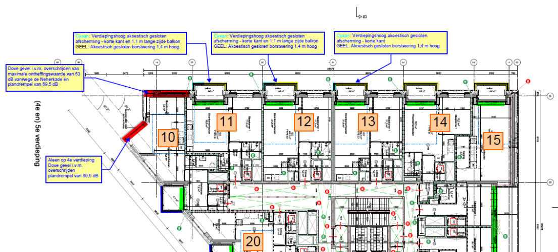
Figuur 2: plattegrond 4 e en 5 e verdieping met nummer appartementen.
