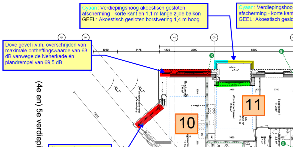
Figuur 4: Balkonscherm bij appartement met nr. 11 meer in detail
