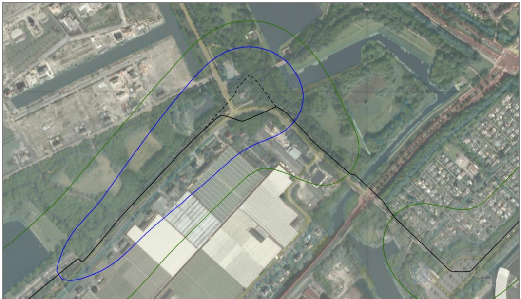
Figuur 3. PR-contouren aardgasleiding W-509-02 nieuwe situatie
