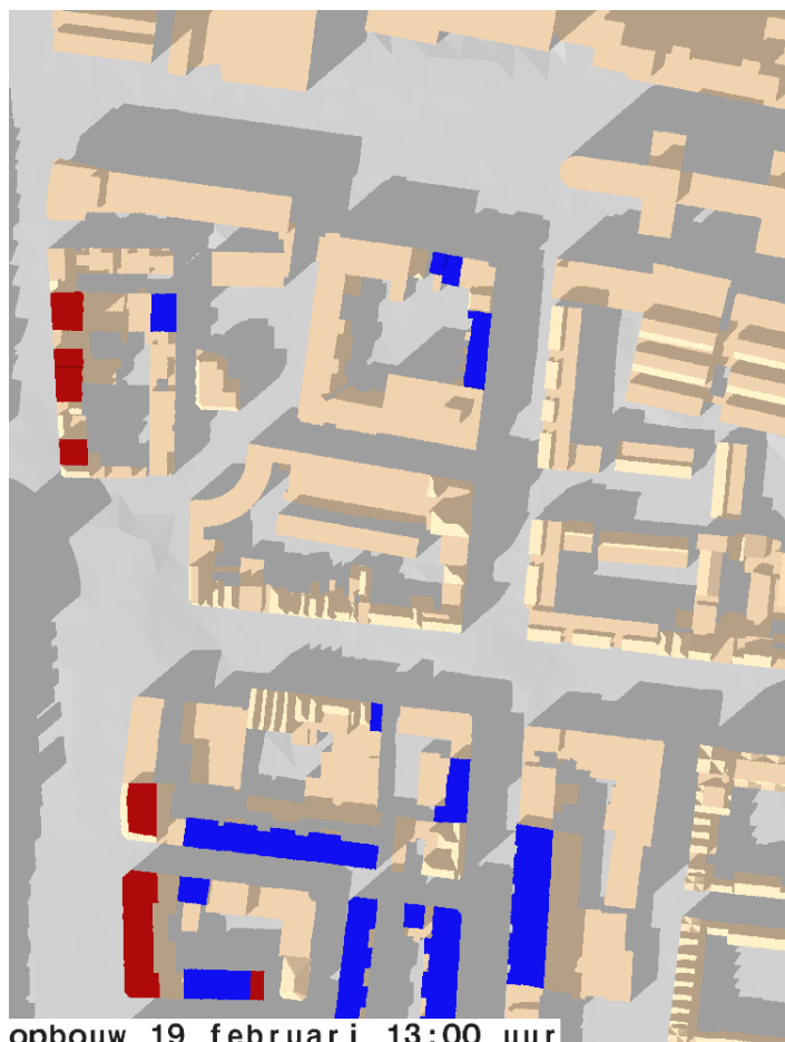
opbouw 19 februari 13:00 uur
