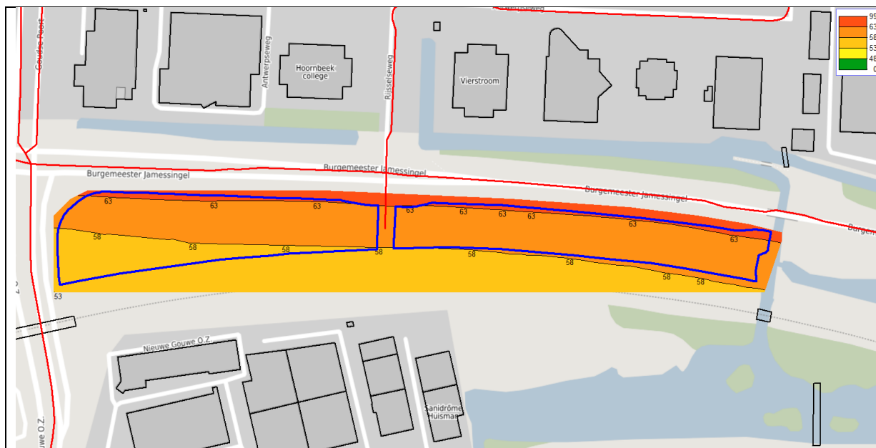
Figuur 7: L_{den} contouren t.g.v. de Burg. Jamessingel incl. aftrek bij DAB
