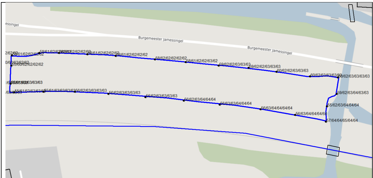
Figuur 18: L_{den} t.g.v.d. spoorbaan t.p.v. bestemmingsvlak A1 oost na toepassen raildempers
