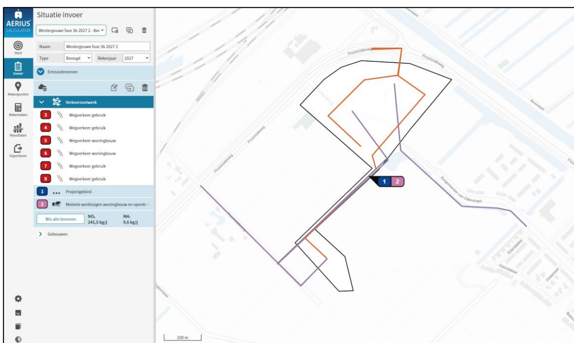
Afbeelding 7. AERIUS-model aanleg- en gebruiksfase 2027
