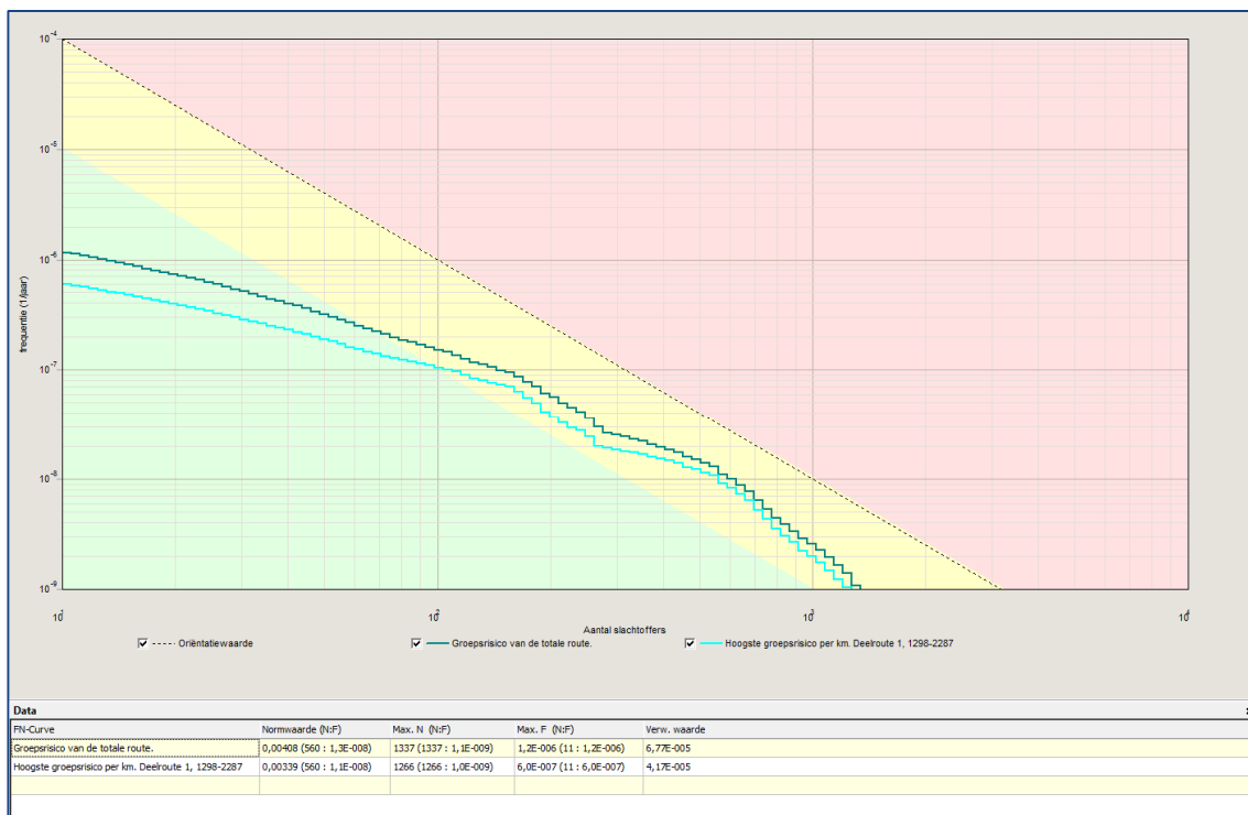
Afbeelding 4 fN-curve berekend groepsrisico, huidige situatie
