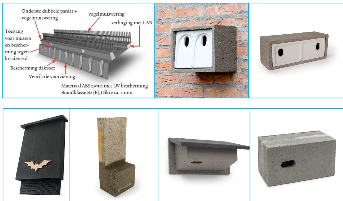
Afbeelding 3: Voorbeelden voorzieningen huismus, gierwaluw en vleermuizen (bron: VivaraPro).
