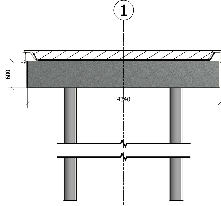
Doorsnede B-B
