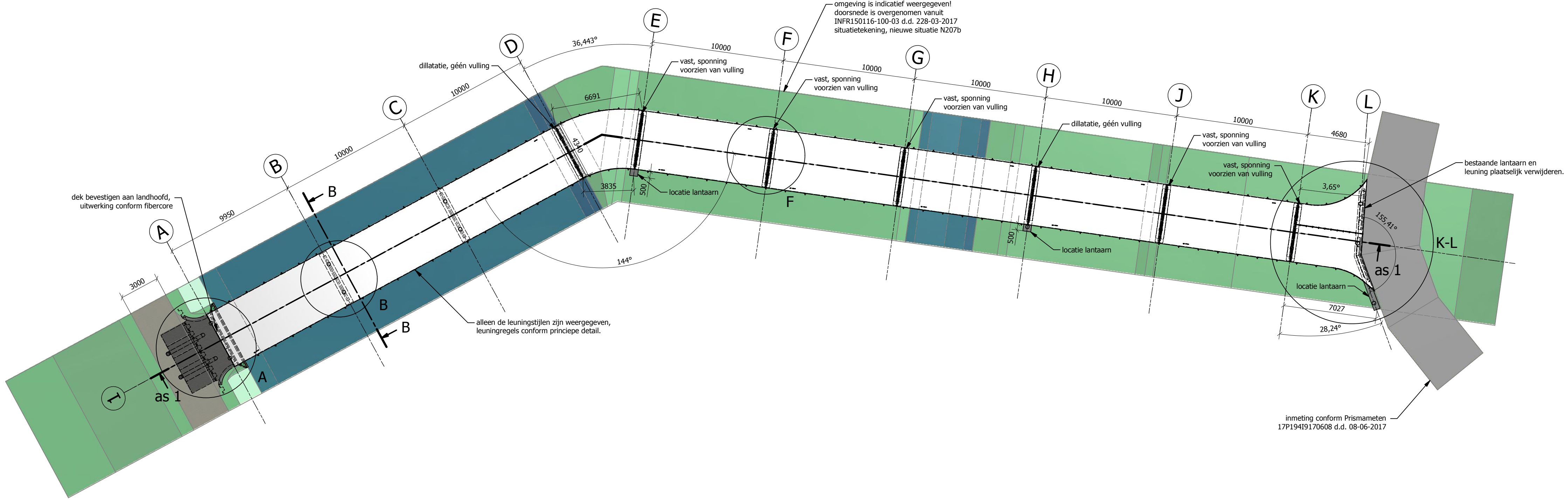
Bovenaanzicht
