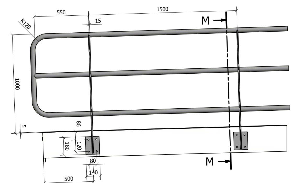
Principe aanzicht leuning
