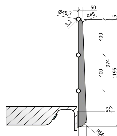
Doorsnede M-M
