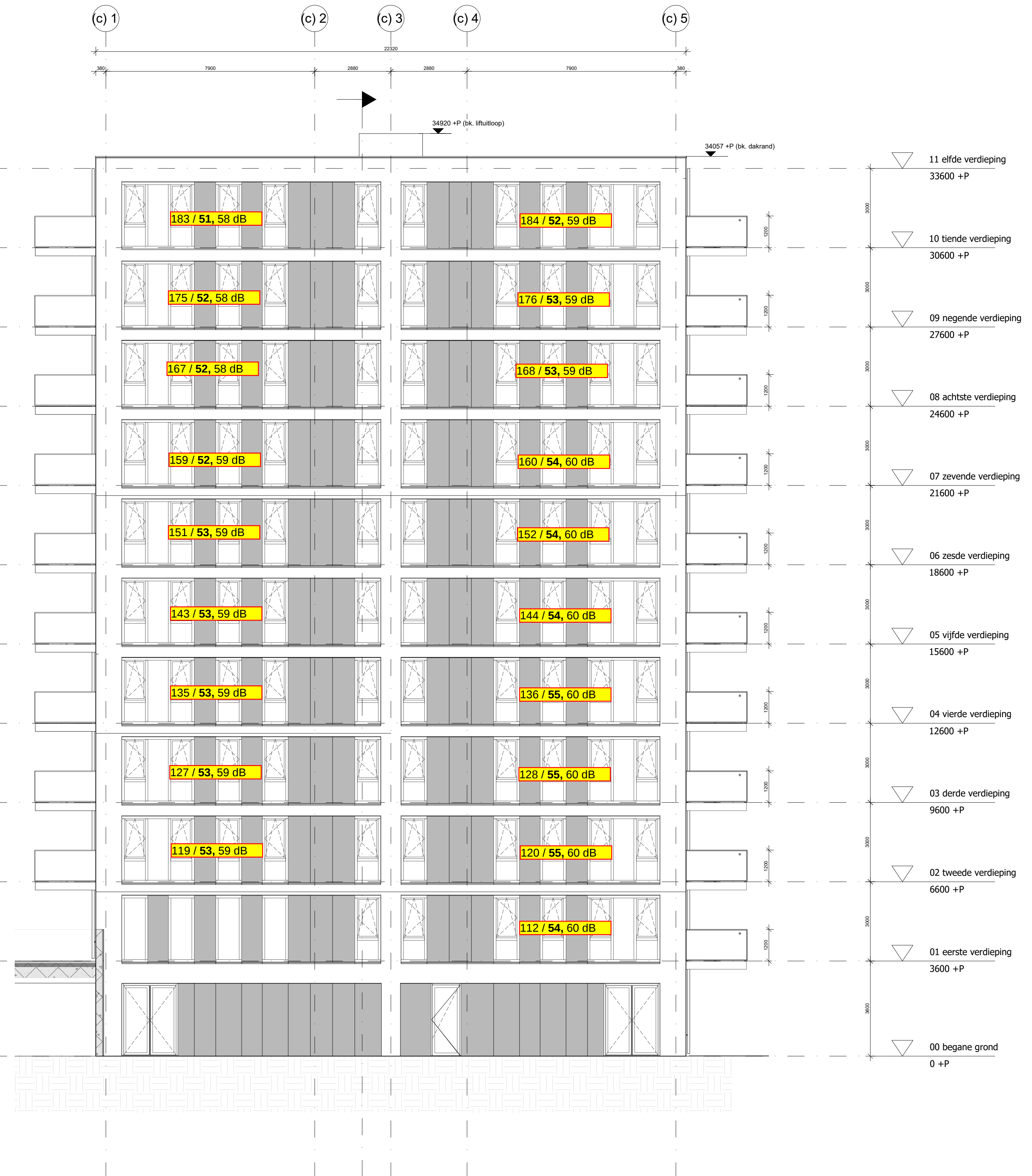
Zuid gevel
