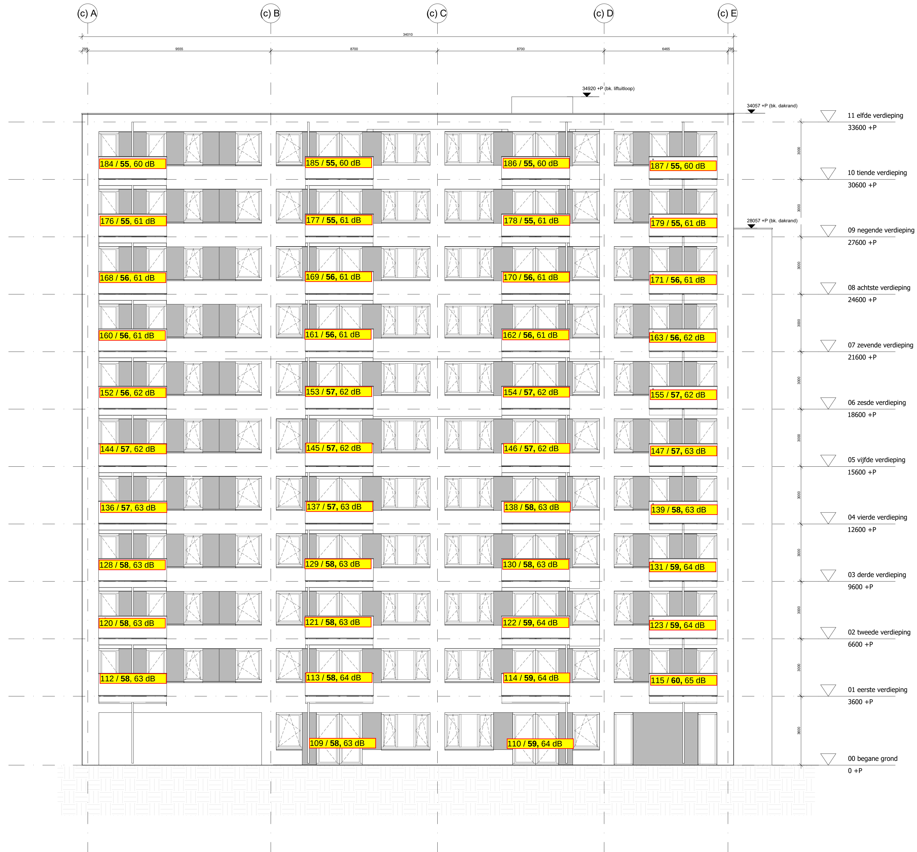
Oost gevel
