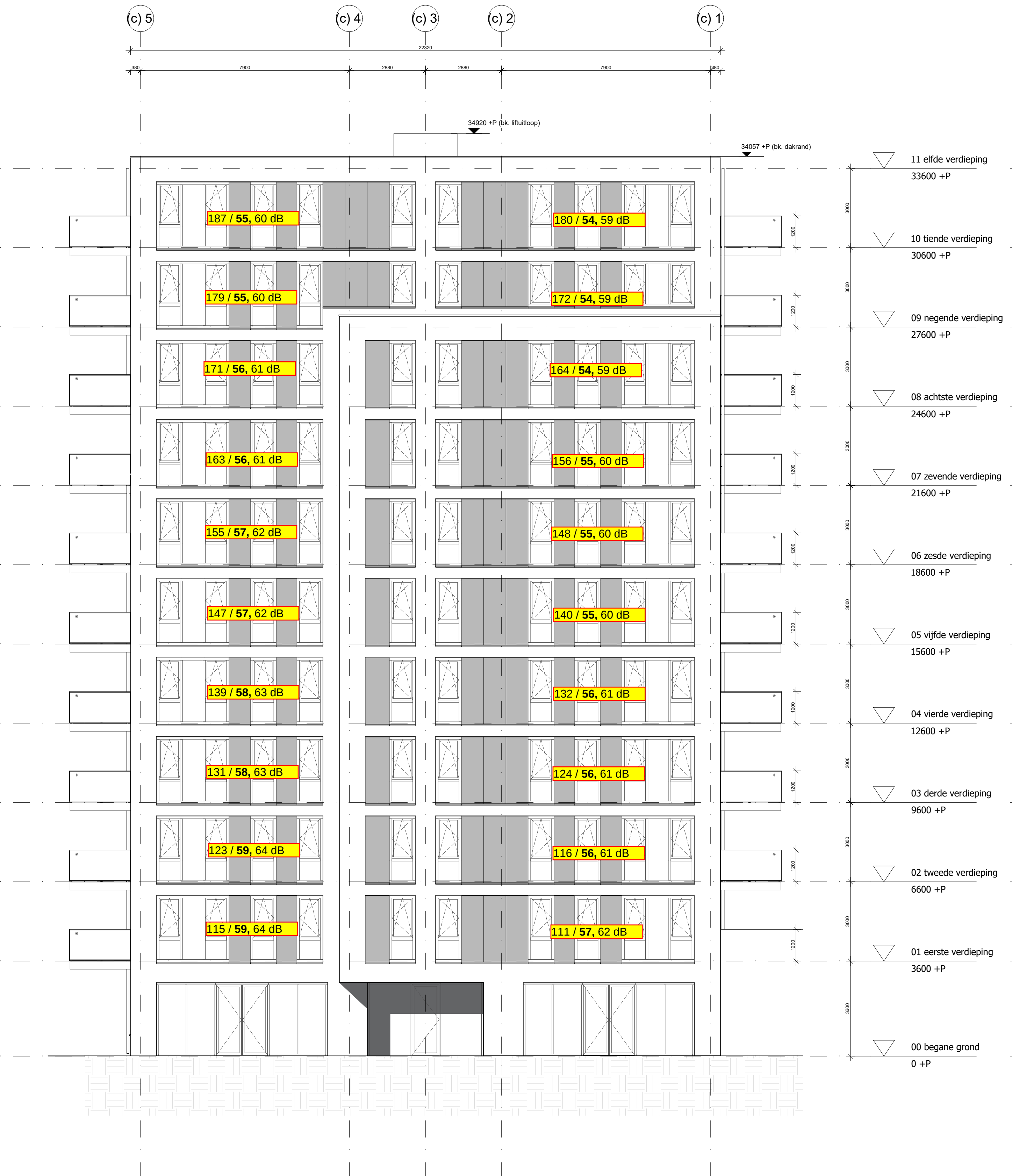
Noord gevel
