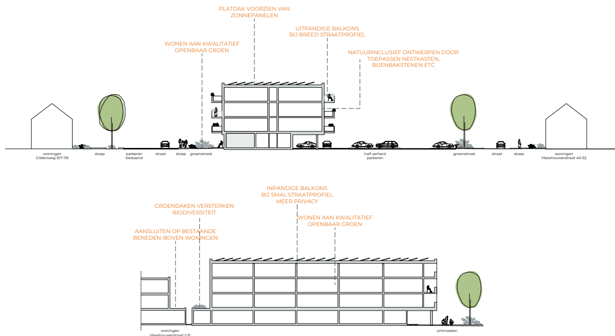
Figuur 3.4: Principedoorsneden toekomstige situatie
